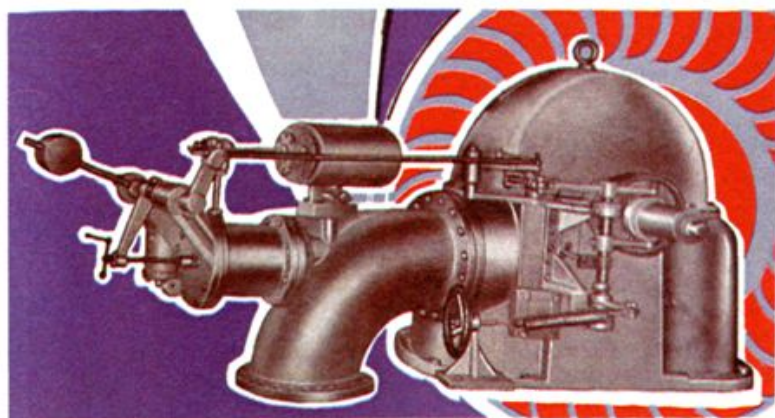
17. 乐清机械厂自行设计生产的水轮机
