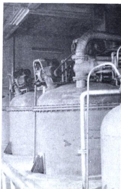
粮油加工工厂精炼车间
