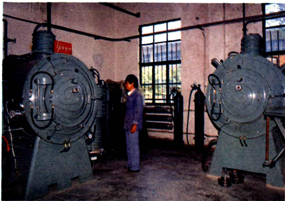
陕西汽车齿轮厂的西德利普森真空淬火回火炉 图2-5
