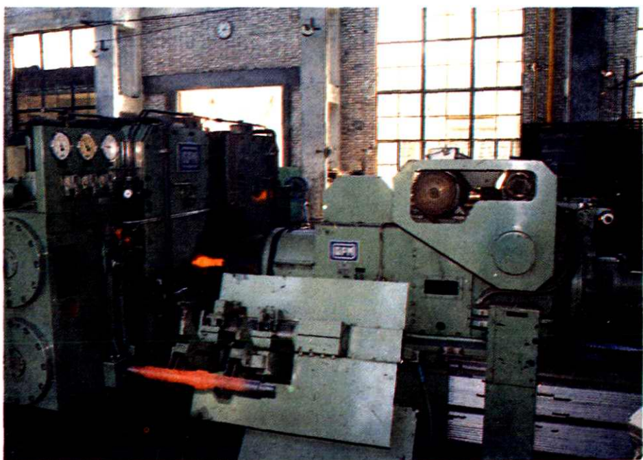
陕西汽车齿轮厂的奥地利精密锻轴机
