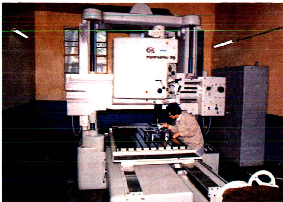
陕西汽车齿轮厂的瑞士光学坐标镗床
