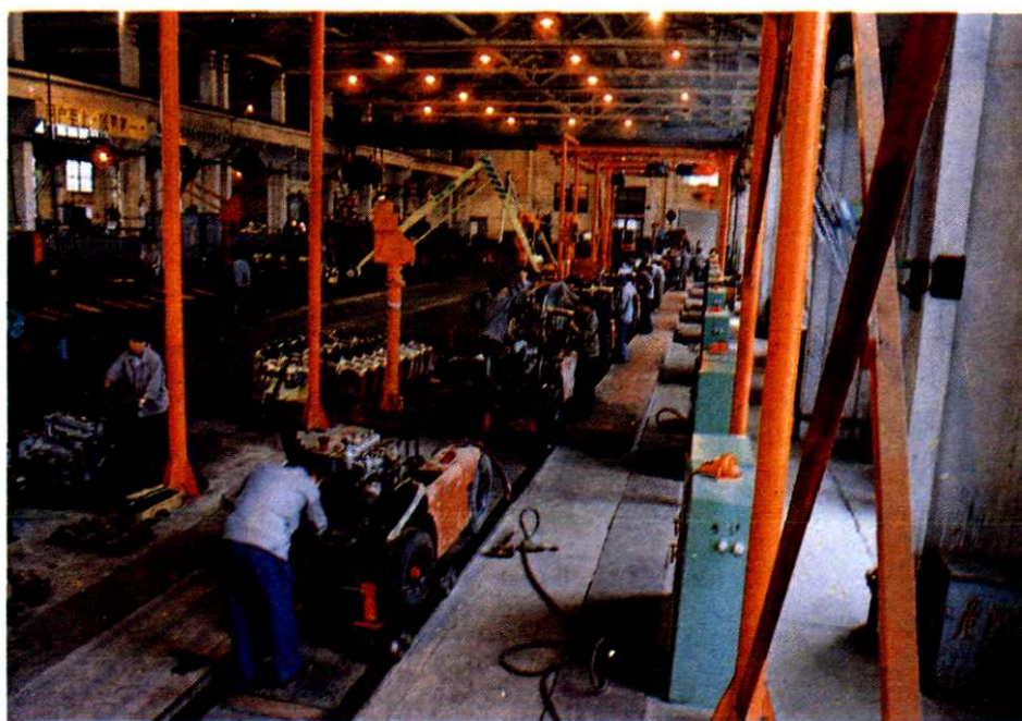
宝鸡叉车制造公司叉车装配自动线 图2-2
