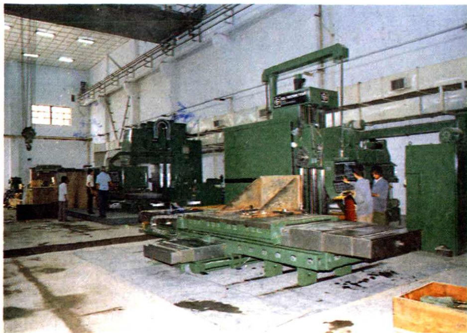
宝鸡石油机械厂引进的数控机床
