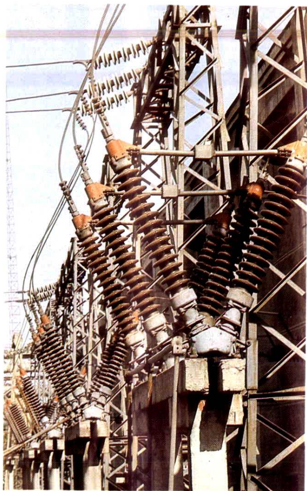
出口线路隔离开关
