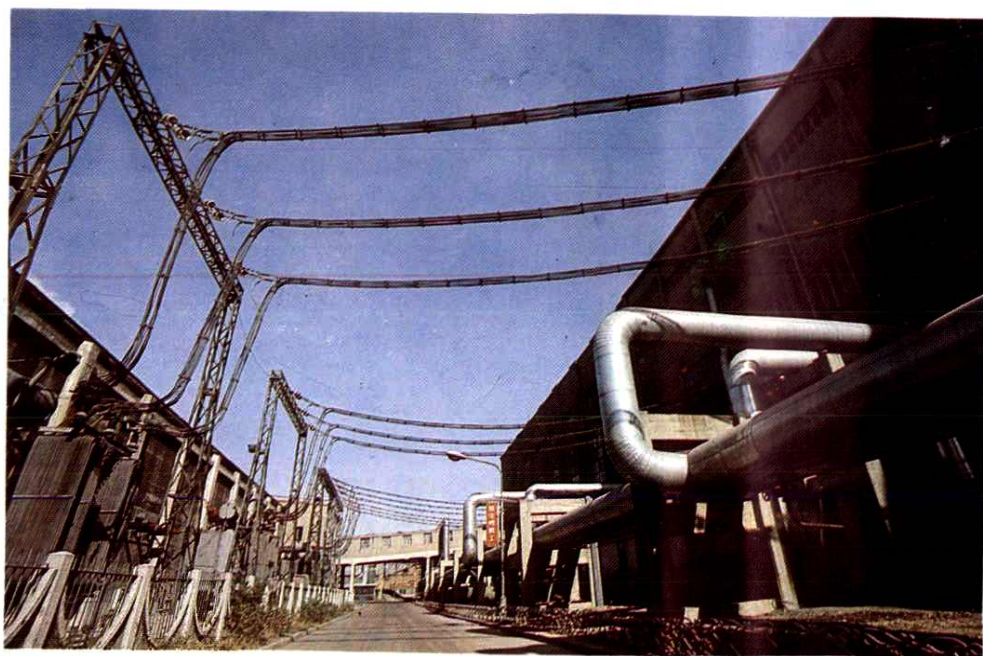
供汽管道与发电机出口引线
