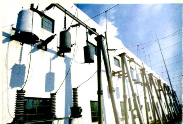
▲ 电气升压站
