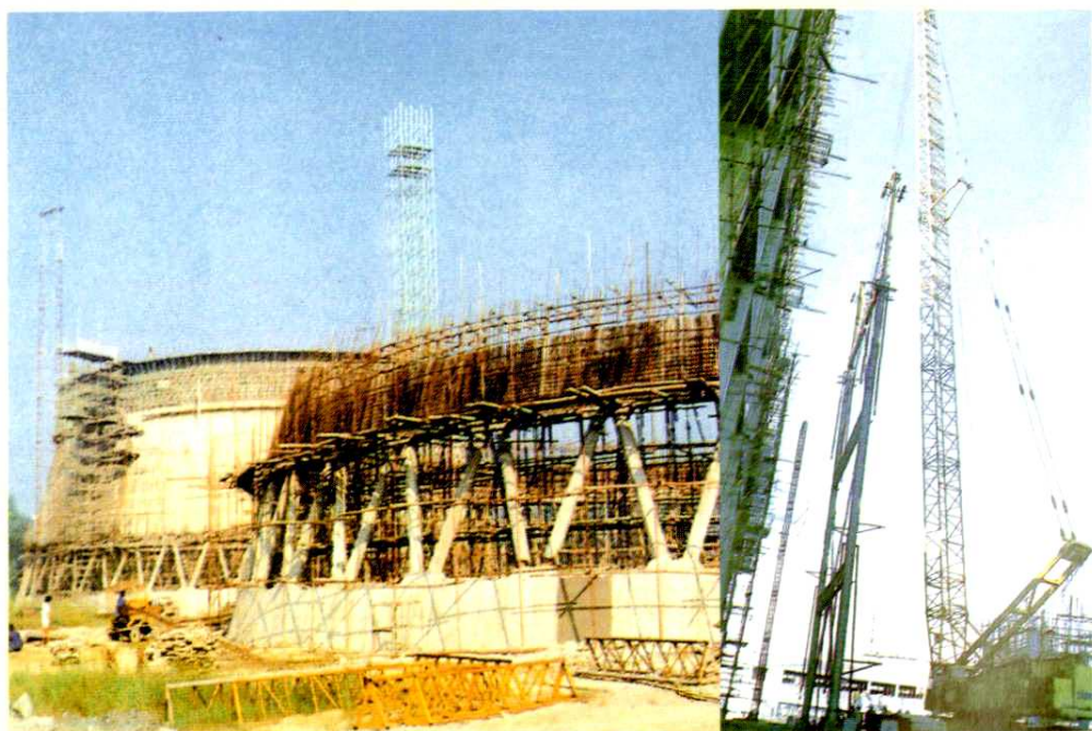
▲ 施工场景
