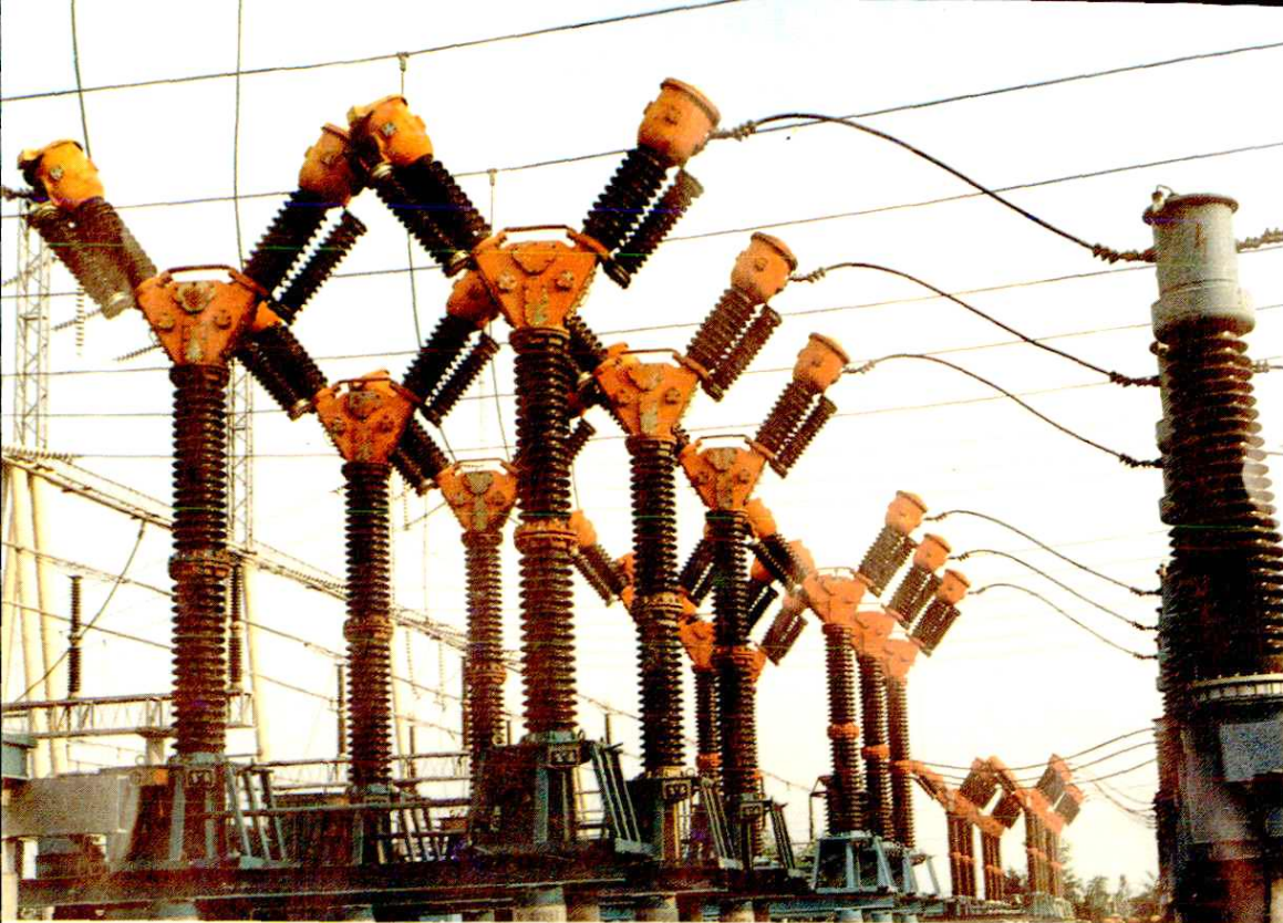
220KV变电站户外设备
