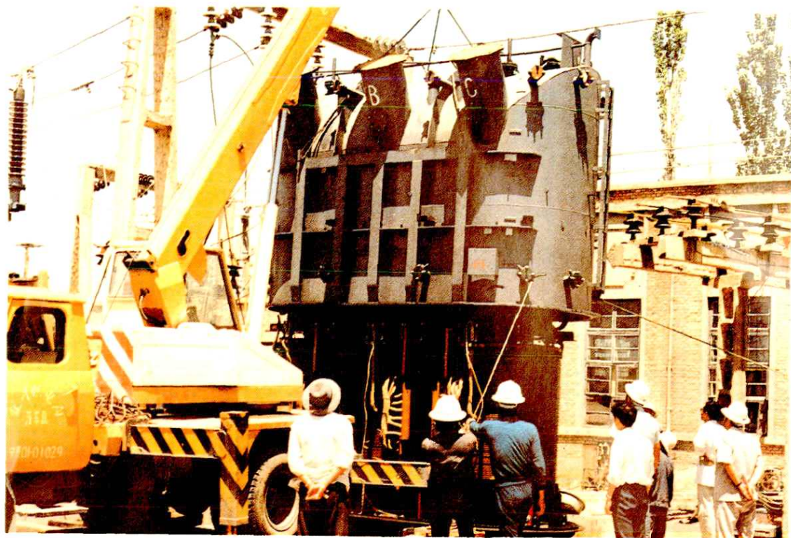
主变压器吊芯检修
