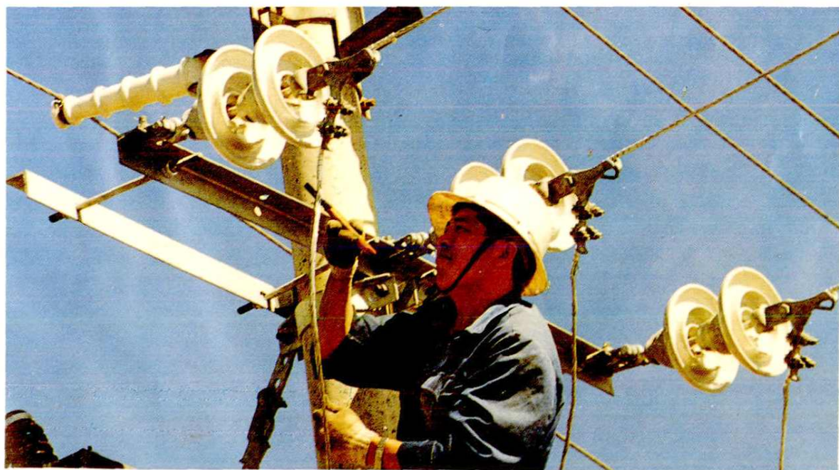
10KV线路检修
