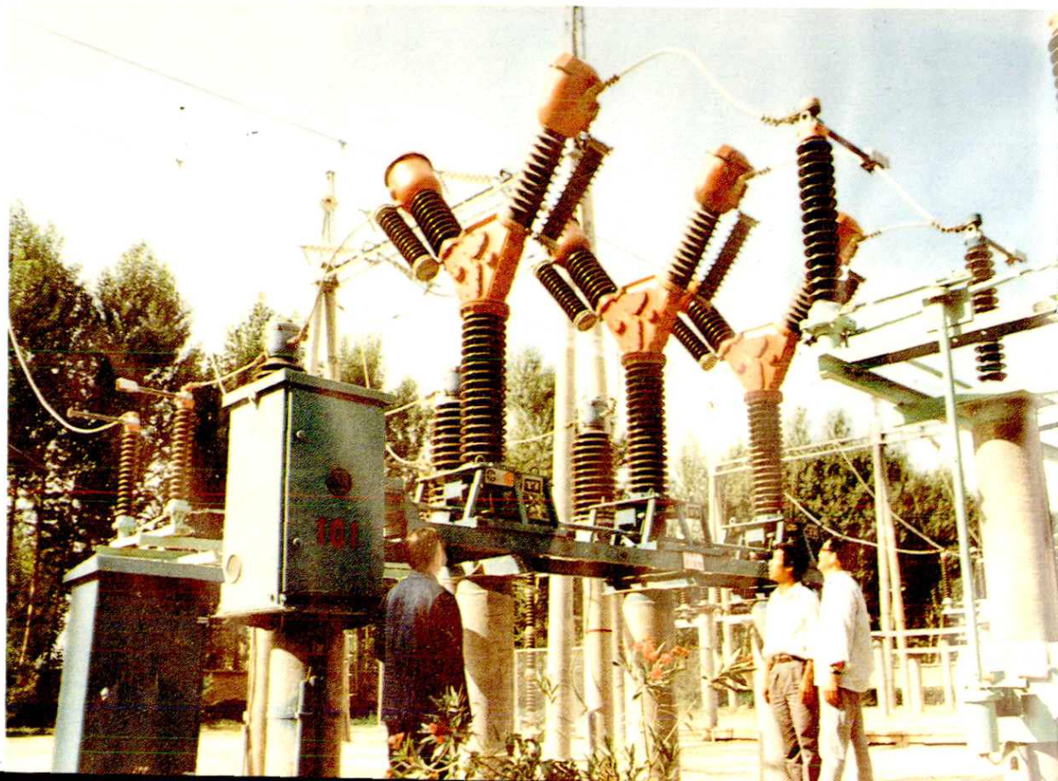
110KV变电站
