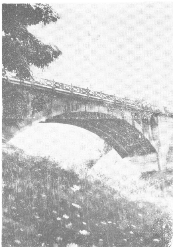
张家渡公路桥于一九七一年十月建成通车
