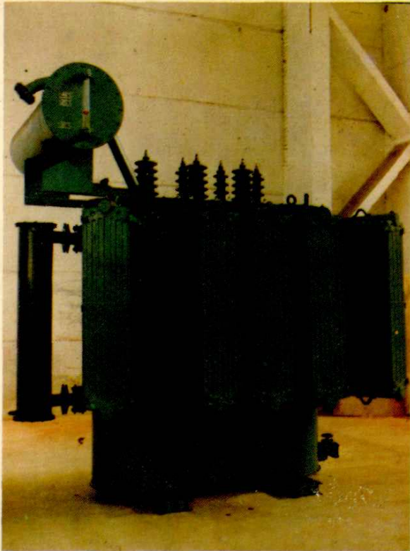
SL7—3150/35 型电力变压器
