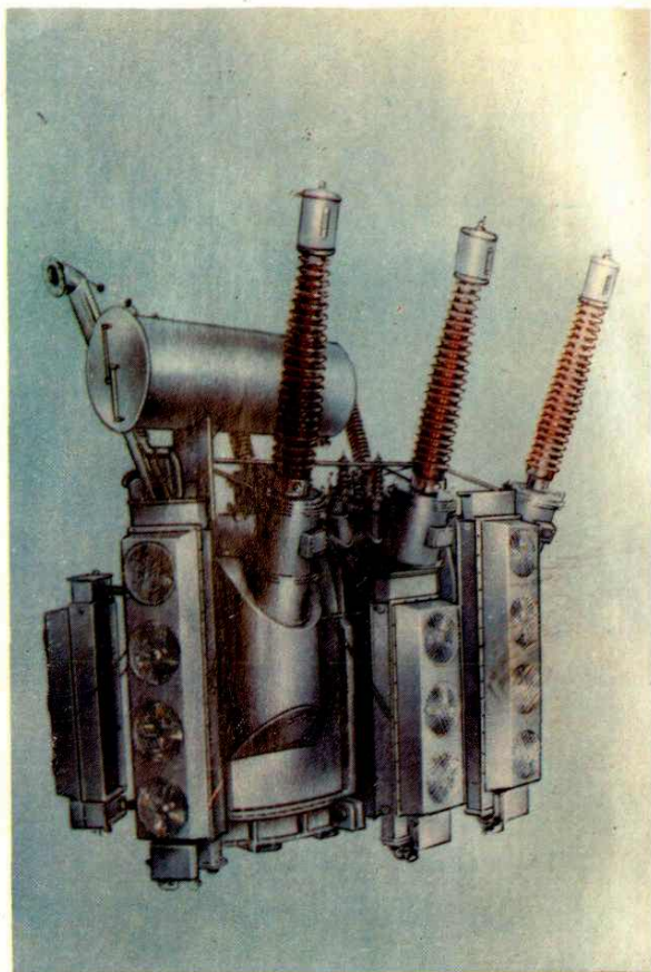
OSFPS—90000/220电力变压器
