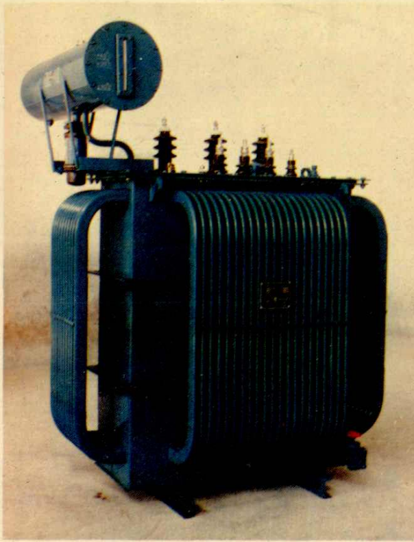
SL7—315/10 型电力变压器
