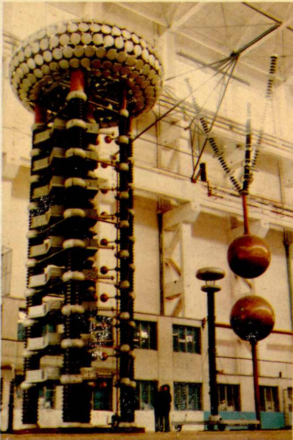
2700千伏冲击电压发生器
