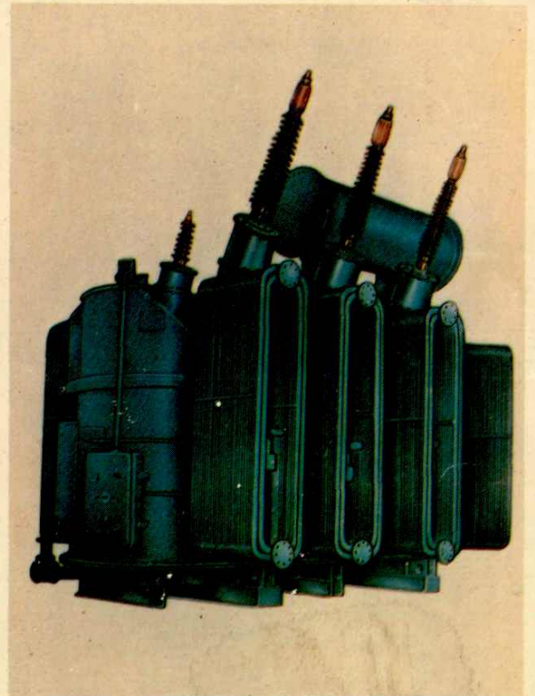
SFSZL7—31500/110 电力变压器
