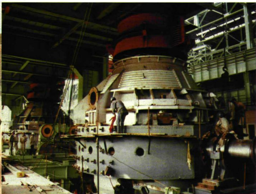
转炉安装
