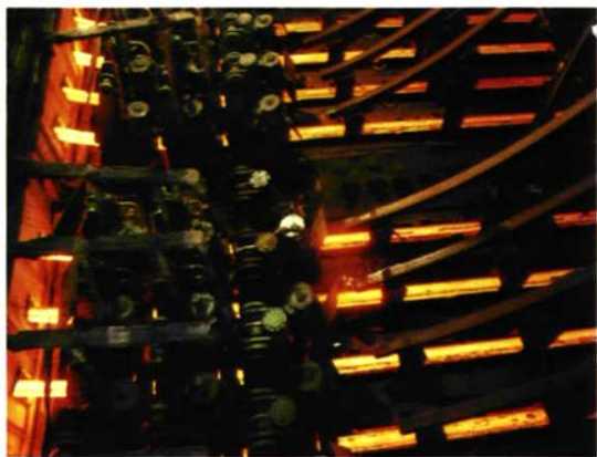
连铸拉矫机
