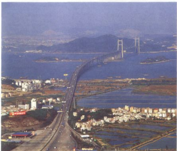
①路堤结合样板工程——沙湾大堤恒联段（1990年摄）
