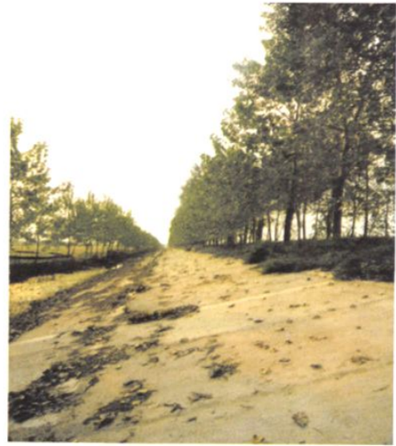
洪泽湖挡洪堤黄圩段混凝土护坡
