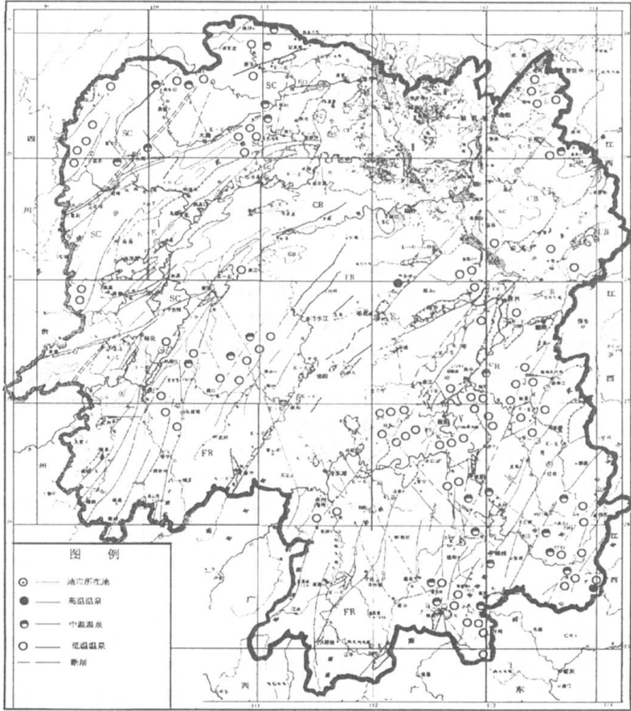
图 1.1.2 湖南省地下温泉分布图
