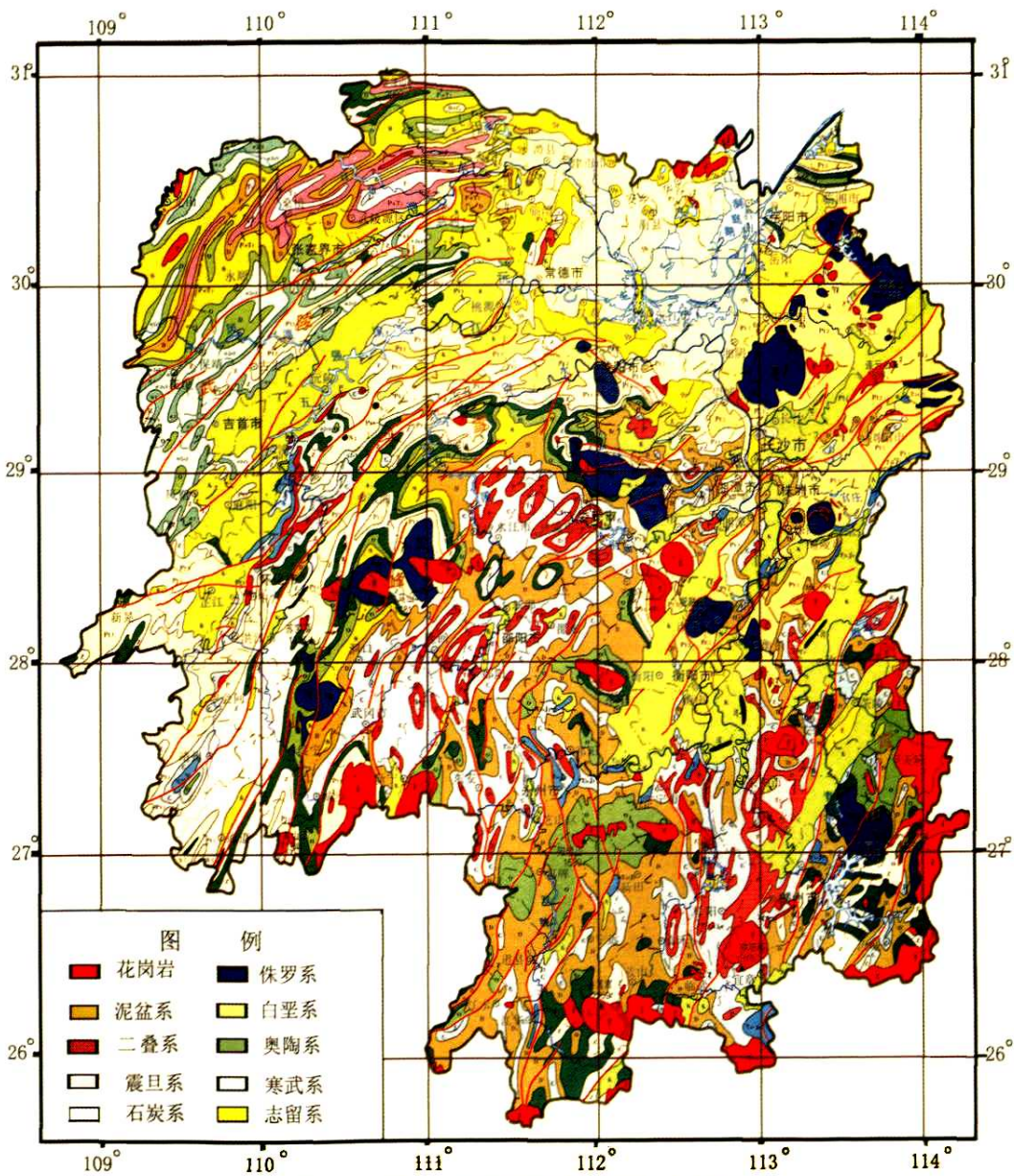
图1.1.1 湖南省地质图(引用《湖南省地图集》)
