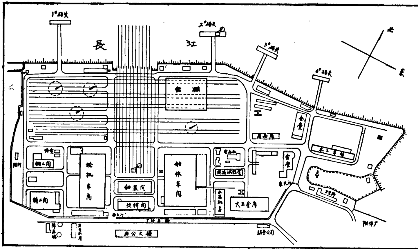
金陵船厂平面图
