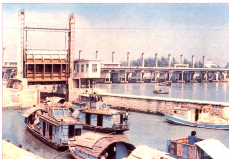
通航 100 吨位的南港船闸
