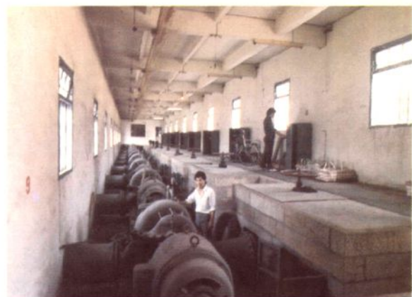
集美抽水机站(9×115 千瓦)
