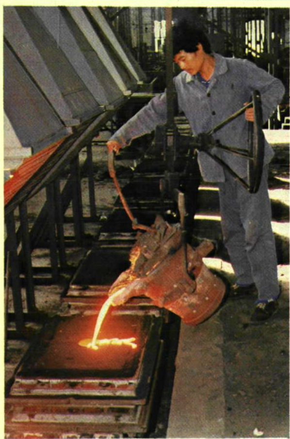
澆鑄自動線
