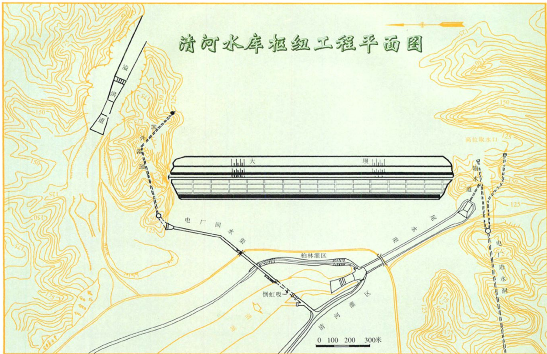
清河水库枢纽工程平面图
