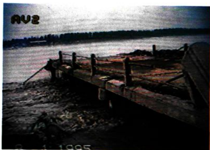
浑河长青桥仅存岸边桥墩
