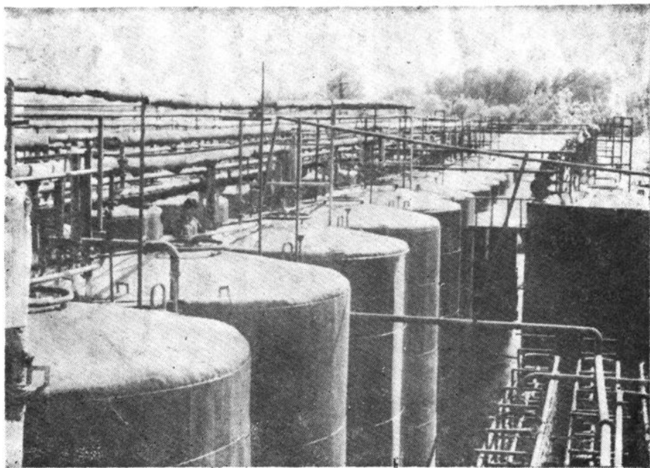
县酒厂酒精发酵罐群
