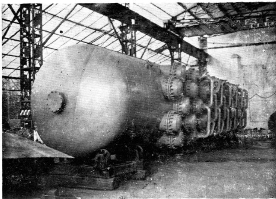
铆焊车间制造的重60吨碳化塔
