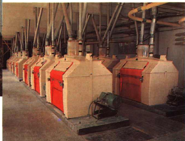
石家庄市等级面粉厂从英国西蒙公司引进的等级面粉生产设备(磨粉机部分)。
