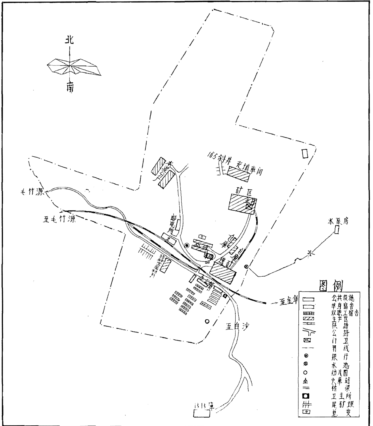
建德铜矿总平面示意图
