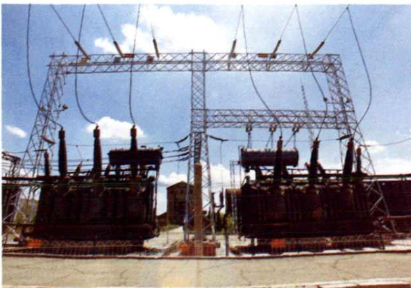
李石寨变电所 2 台 18 万千伏安主变压器
