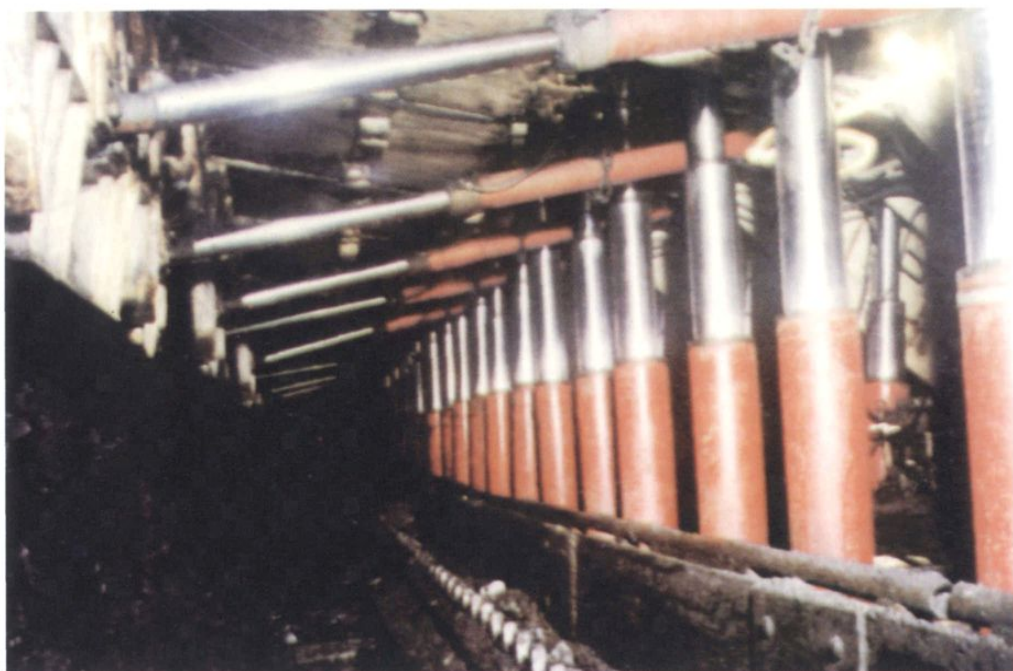
普通综采工作面
