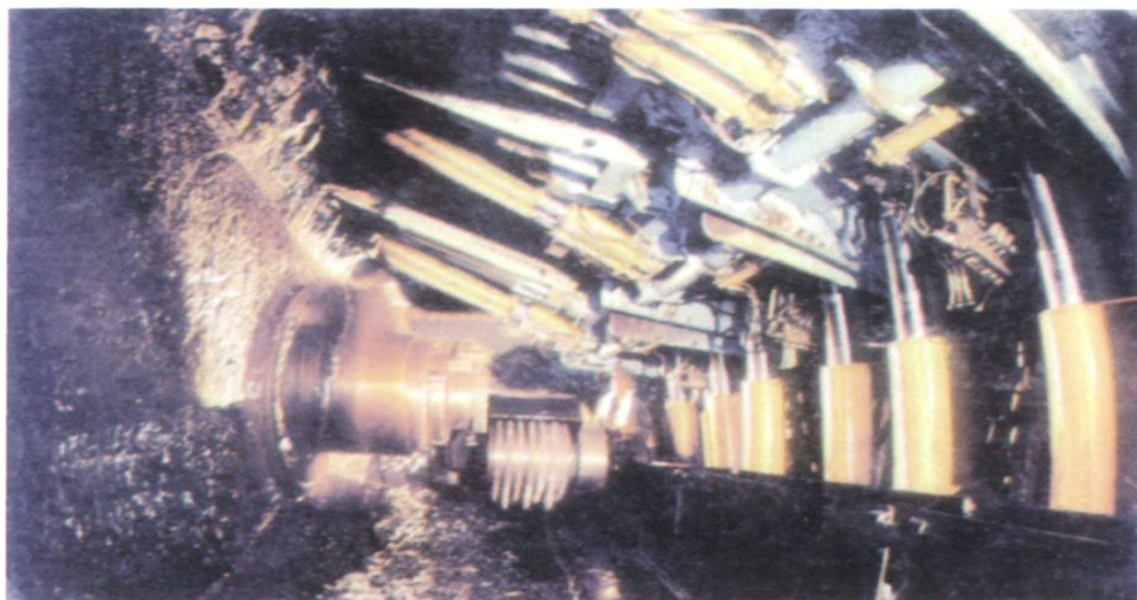
放顶煤综采工作面
