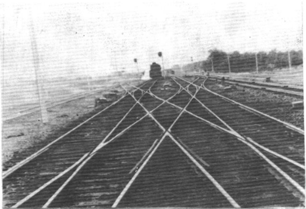
商丘西运转场复式交分道岔
