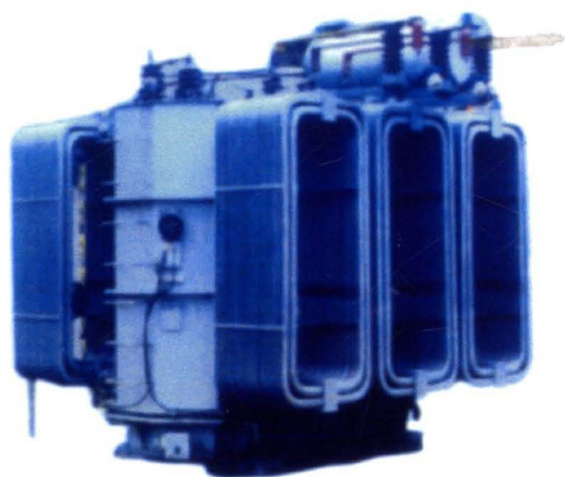
长征电器公司生产的电力变压器
