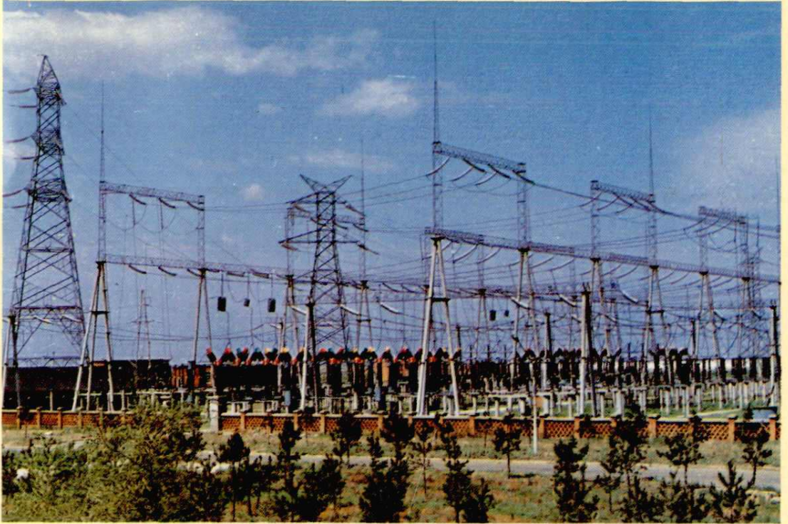
220 千伏开关场一角
