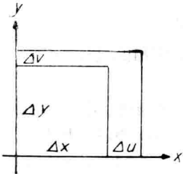
图 1.7 正应变和位移的关系
