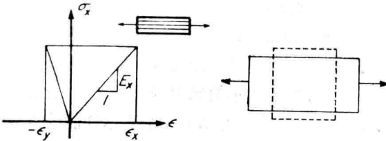
图 1.11 纵向单轴拉伸试验。正方形变成矩形
