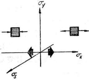
图 1.3 拉伸和压缩时纵向单轴应力。各单位矢量是 (\pm 1, 0, 0)
