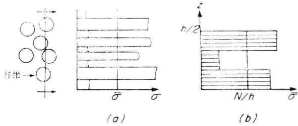
图 1.1 局部应力和平均应力之间的示意关系 (a) 微观力学标准的模型, 可分辨出纤维和基体中的应力。这应力平均值就是铺层应力。 (b) 宏观力学标准的模型, 可分辨出铺层和铺层组的应力。这应力平均值就是层合板应力
