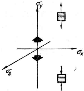
图 1.4 拉伸和压缩时横向单轴应力。各单位矢量是 (0, \pm 1, 0)
