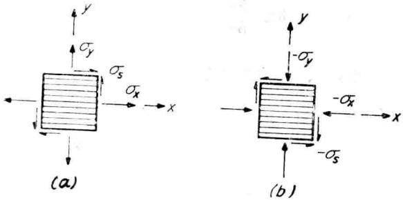
图 1.6 应力分量的符号规则 (a) 给出的所有分量为正， (b) 给出的所有分量为负
