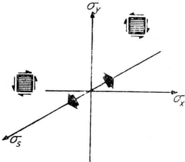
图 1.5 正、负纵向剪切。各单位矢量是 (0, 0, \pm 1)
