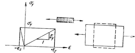
图 1.12 横向单轴拉伸试验
