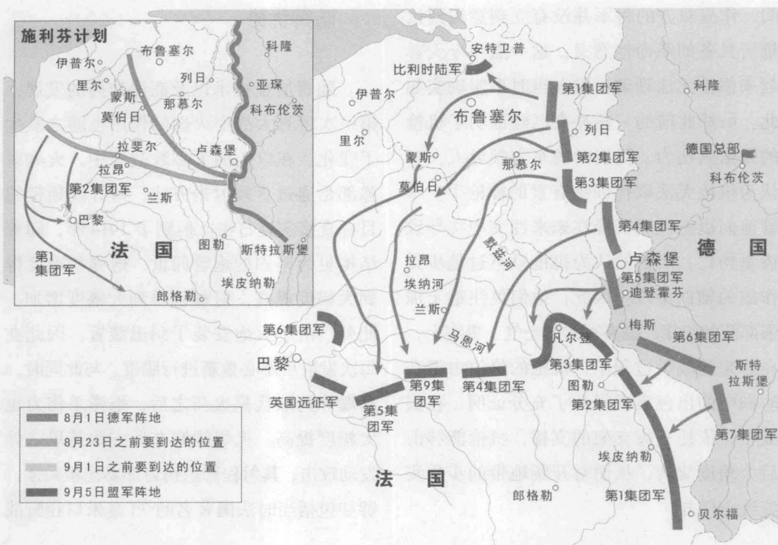
上图：德国战前制订的入侵比利时和法国的“施利芬计划”示意图（左上角），以及战时的战局进展示意图。一战爆发后，德军右翼部队未能实现包围巴黎的预订计划。
