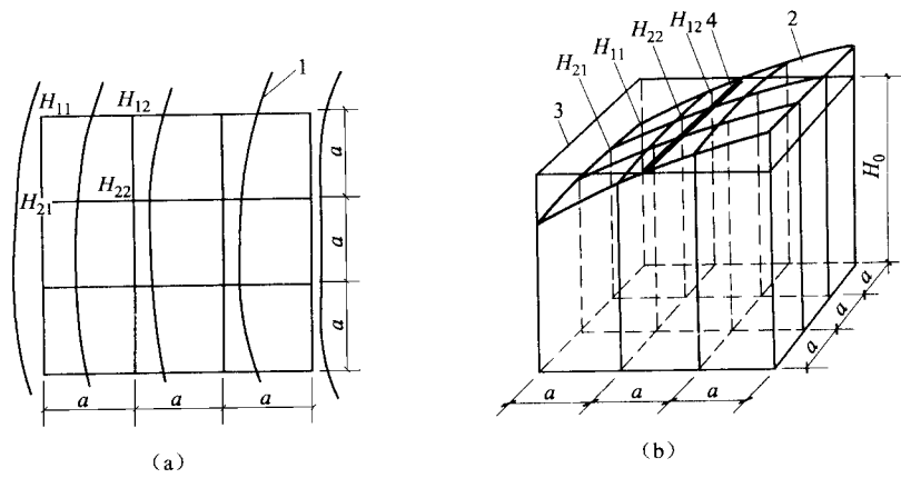
图 1-2 场地设计标高计算简图
