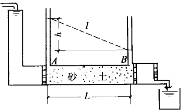
图 1-1 砂土渗透实验
