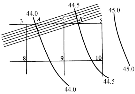
图 1-3 内插法的图解法
