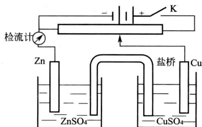
图 1-2 Cu-Zn 电解池示意图
