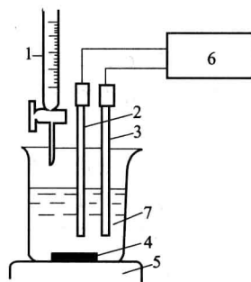
图 1-4 电位滴定示意图
