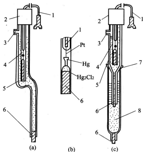
图 1-5 甘汞电极
