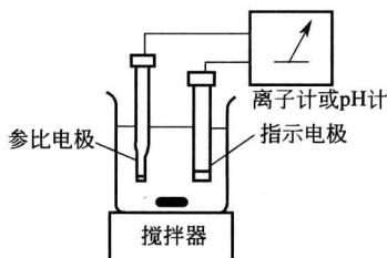
图 1-3 直接电位法示意图
