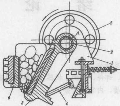
图2 颚式破碎机
