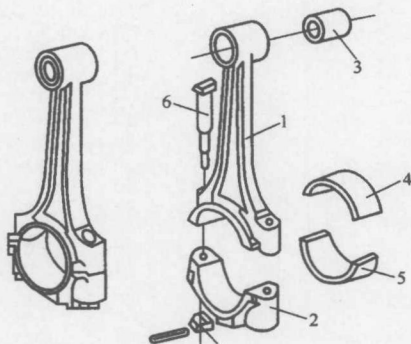
图4 连杆简图
