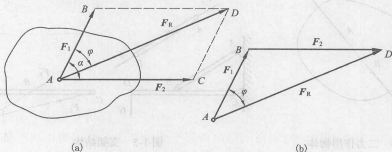
图 1-7 力的合成
