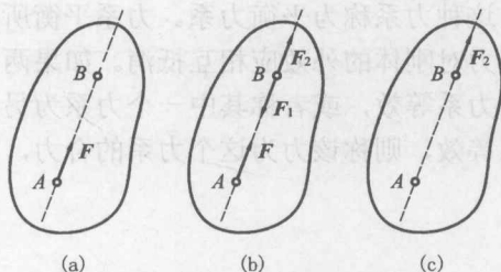
图 1-6 力的传递
