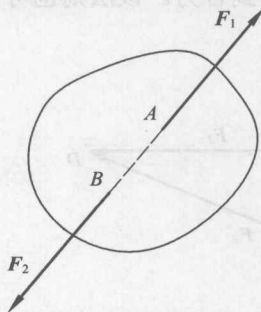
图 1-4 二力作用物体
