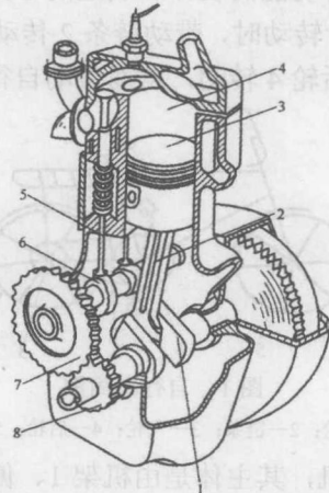
图3 单缸内燃机
