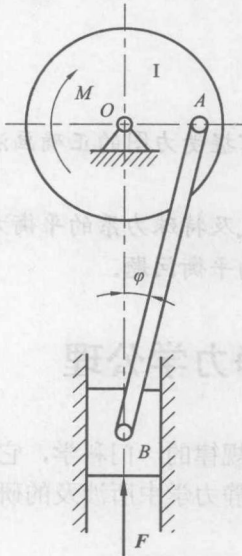
图 1-1 曲柄滑块机构
