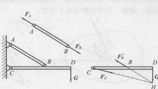
图 1-5 支架结构
