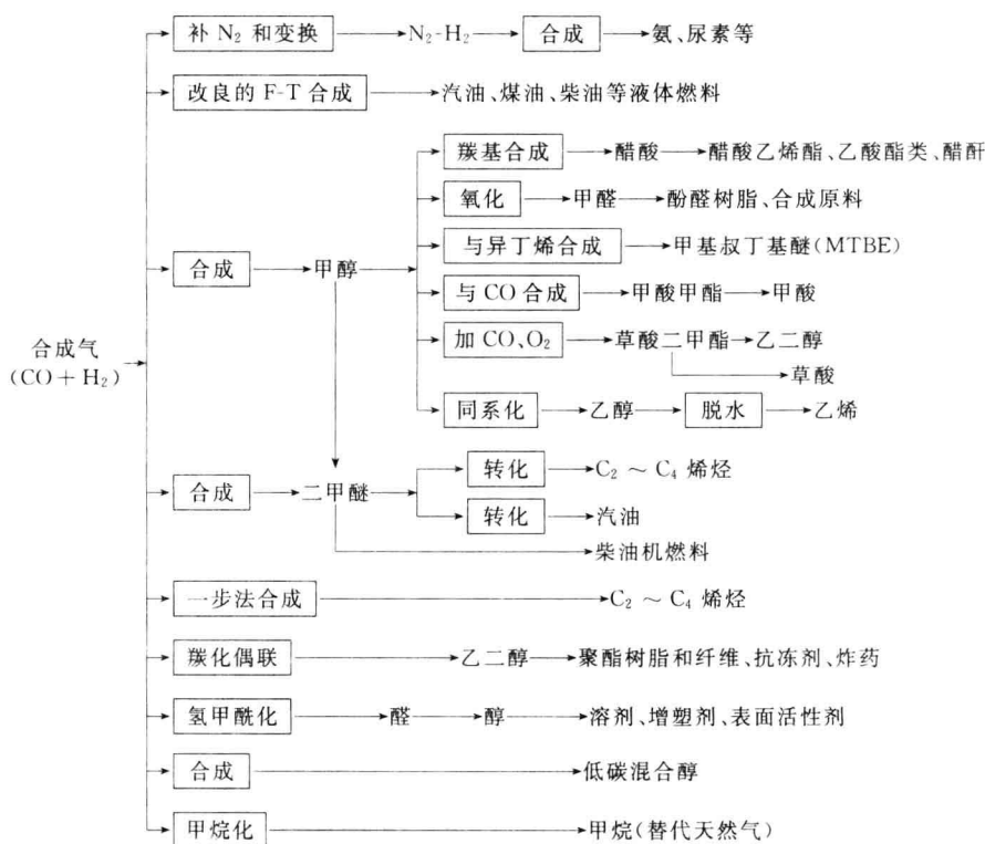
图 1-8 以合成气为原料生产的主要化工产品
