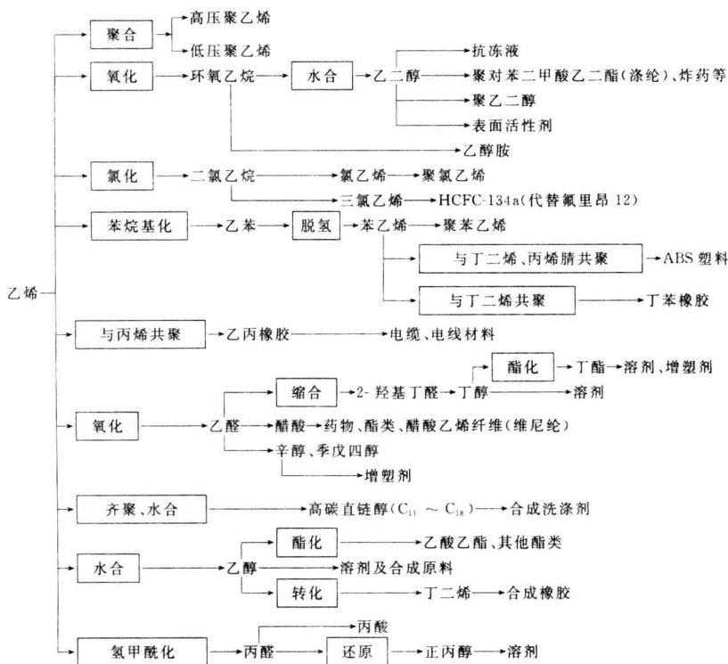
图 1-3 以乙烯为原料生产的主要化工产品
