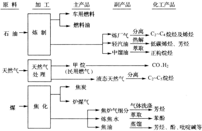
图 1-2 由石油、天然气、煤加工副产物所得化工产品
