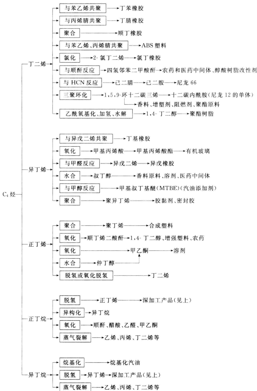
图 1-5 以 C 4 烃类为原料生产的主要化工产品
