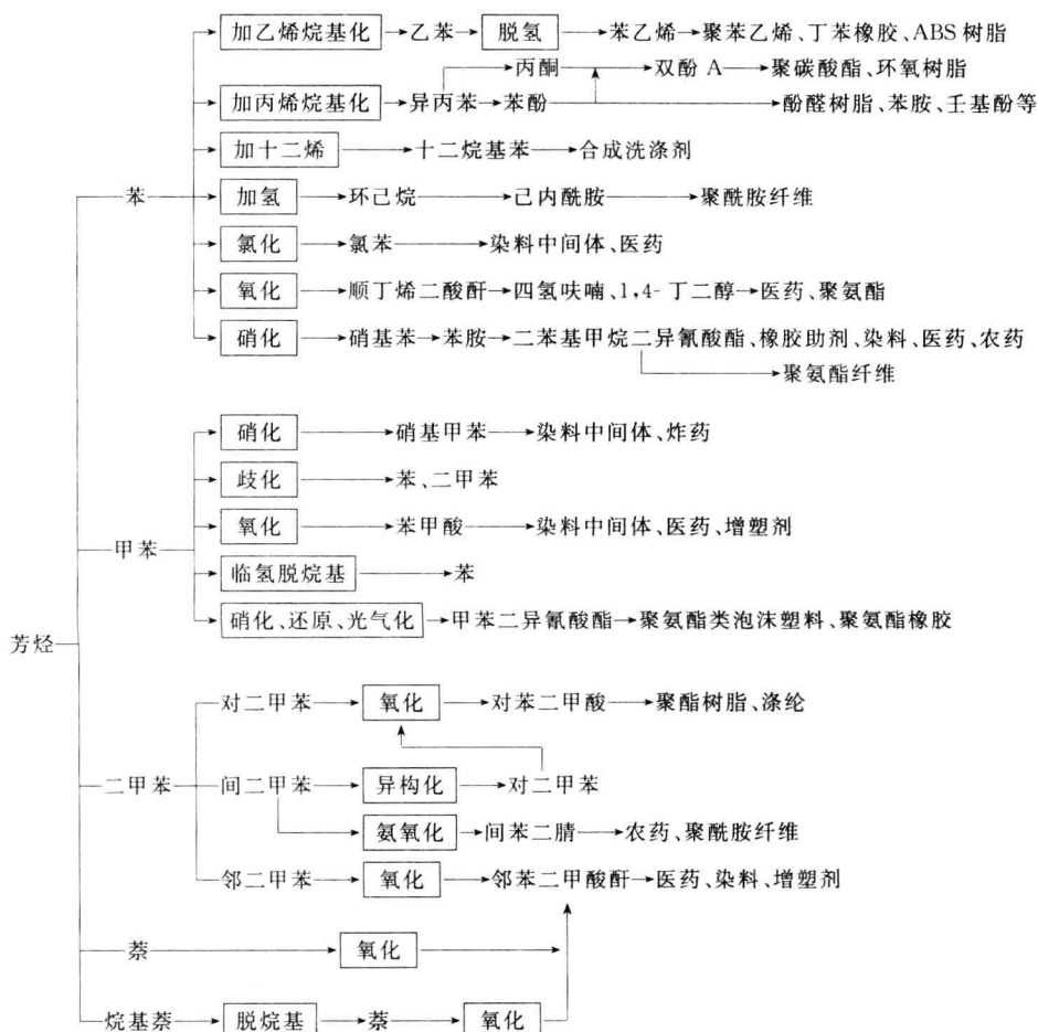
图 1-6 以芳烃为原料生产的主要化工产品
