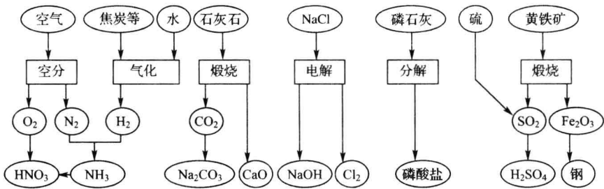
图 1-1 无机化工的重要原料
