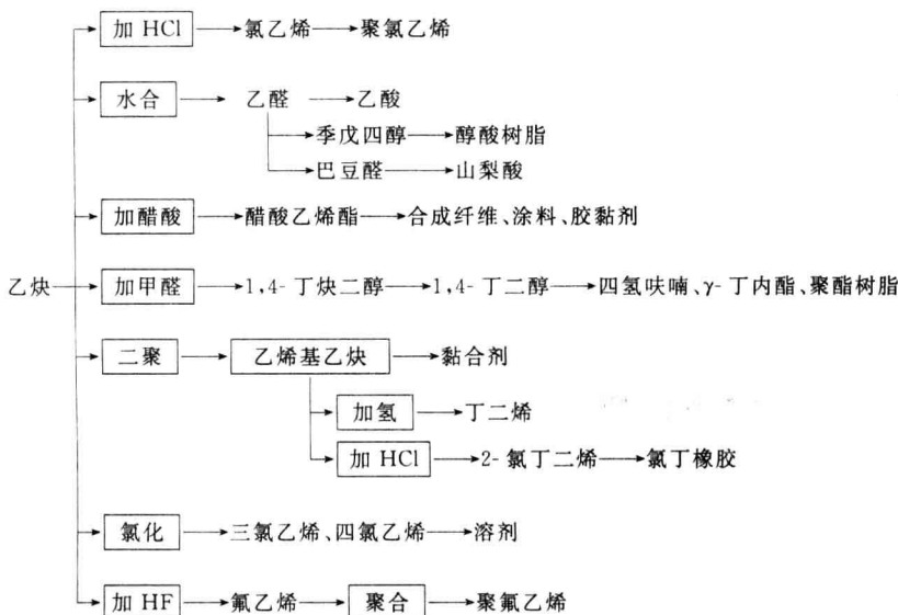
图 1-7 以乙炔为原料生产的主要化工产品
