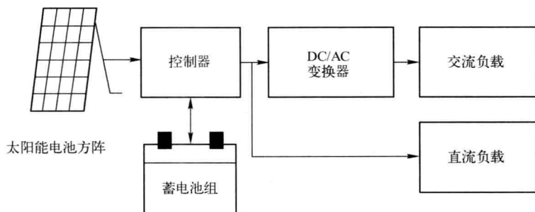
图 1-2 独立太阳能光伏系统构成
