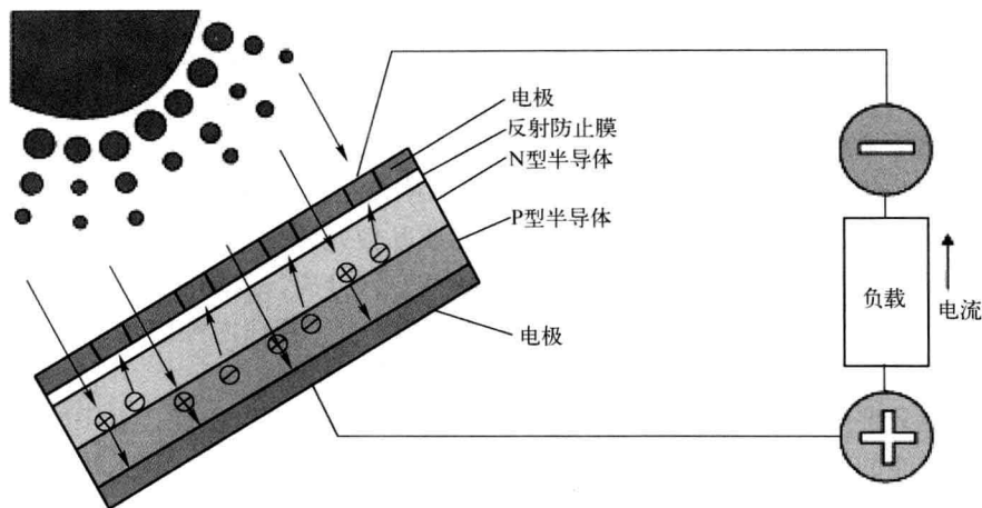
图 1-1 太阳能光伏发电原理
