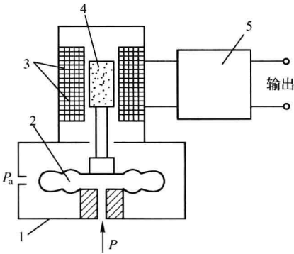
1—固定连接；2—膜盒；3—电感线圈；4—磁芯；5—转换电路 图 1.3 压力传感器示意图
