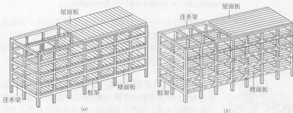
图 1-3 纯框架体系示意
