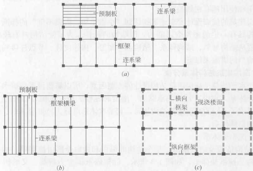
图 1-4 纯框架体系分类 (a) 横向框架承重; (b) 纵向框架承重; (c) 纵横向框架承重
