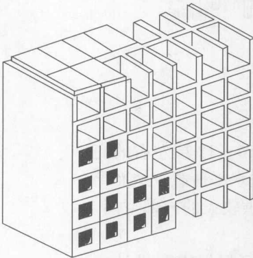
图 1-5 纯剪力墙体系示意
