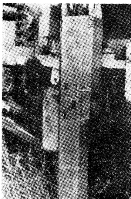
图 1 自动钻进式横向触探仪，水平探头在向仪器内退缩
