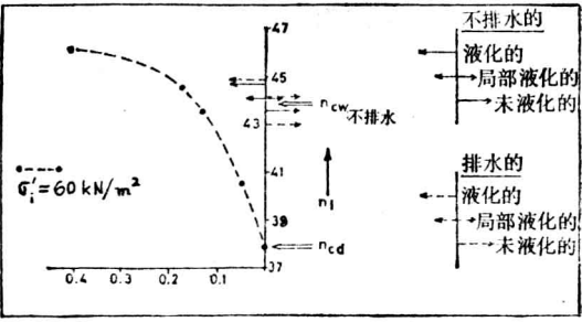
图2 包括试样1的湿临界密度试验成果的干试验的 \varepsilon_{vol_{max}} 与 n_i 图
