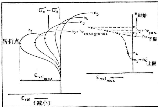
图 1 按 Casagrande 和 Geuze 的临界密度
