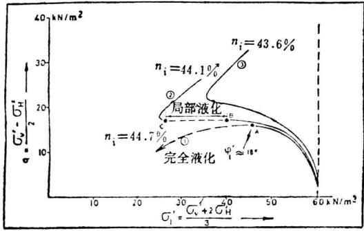
图3 对试样1的三个湿临界密度试验的各种应力途径
