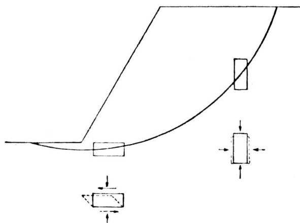
图 1 室内抗剪强度与野外抗剪强度的对比
