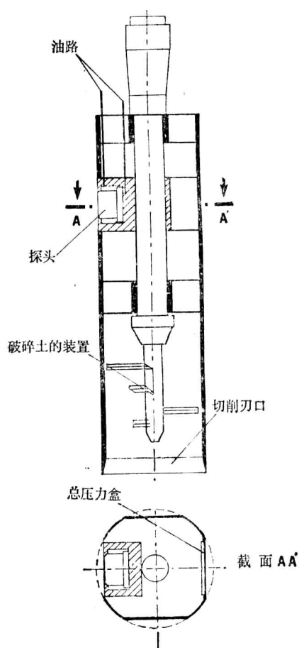
图 2 自动钻进式横向触探仪工作原理简图
