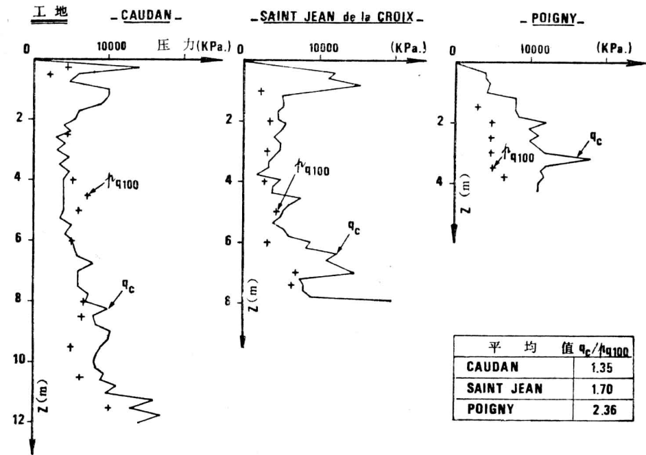
图 5 当相对变形为100%时，圆锥阻力 q_c 与水平贯入强度 p_q 的比较
