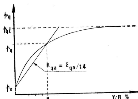
图 3 典型的水平贯入试验曲线。所测得诸特征值的定义
