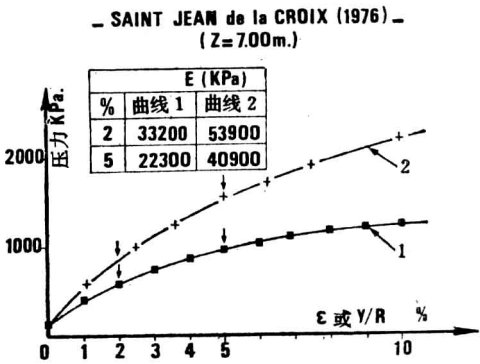
图 4 ST-JEAN-DE-LA-CROIX 工地。自动钻进式旁压仪与自动钻进式横向触探仪所测得应力-应变曲线的比较
