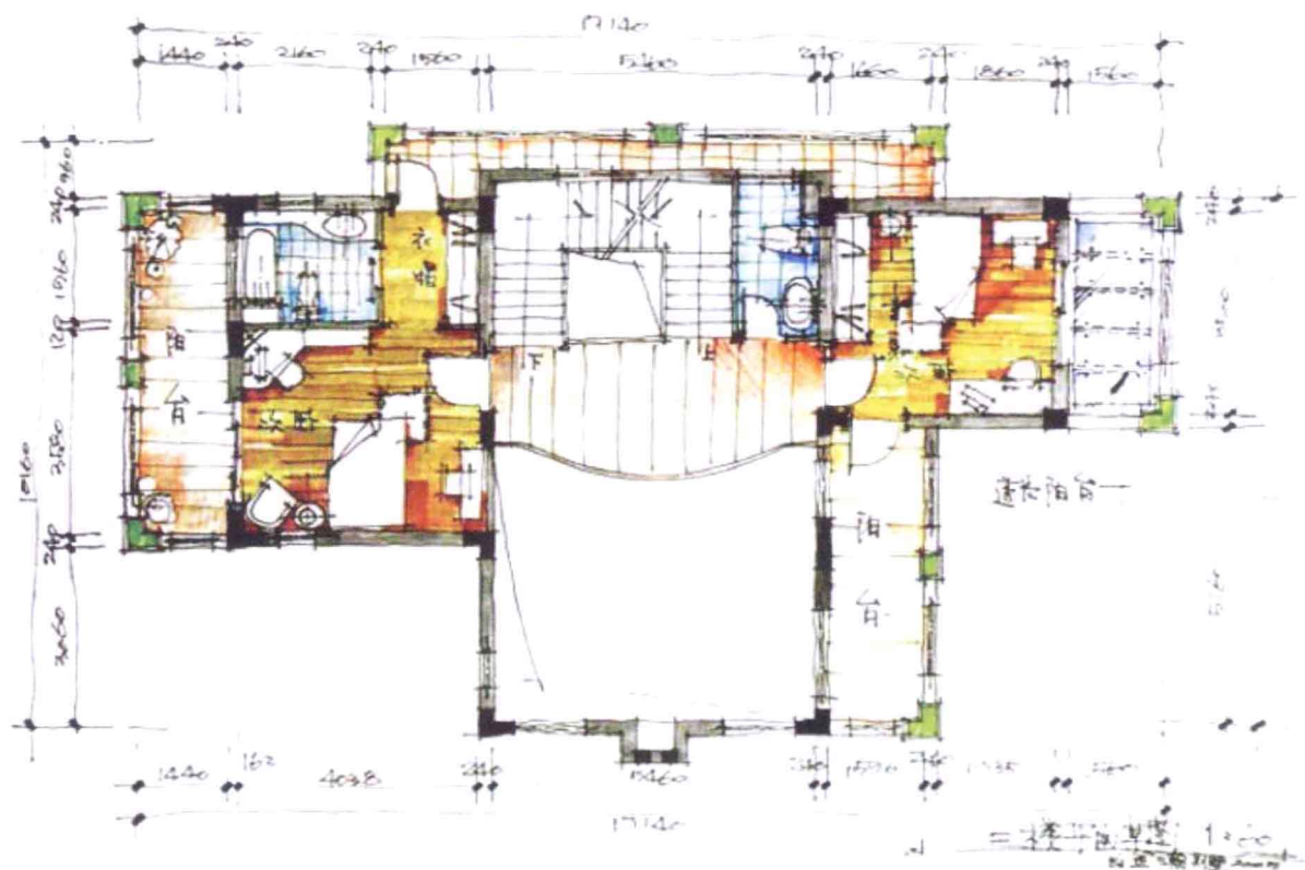
图1-5 手绘平面图即使不够精彩也无关系，只要能表达出主要设计内容和简单色彩就可以了。
