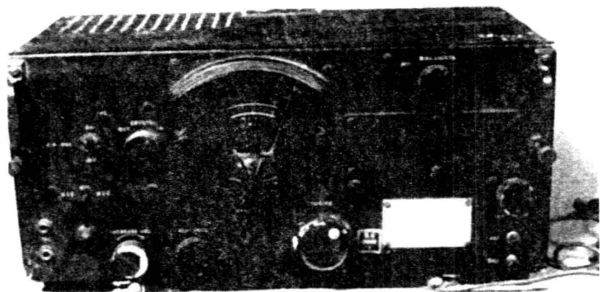
1937年在上海使用的与共产国际联络的发报机
