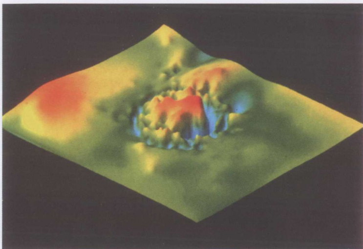
彩图 10. 奇克苏鲁布地区的异常磁场透视图。[加拿大地质调查局皮尔金顿(Mark Pilkington)特许翻印]
