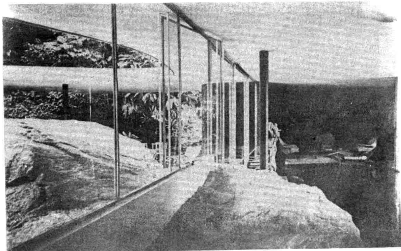
Oscar Niemeyer 設計之自宅(1942年位於巴西·里約熱內盧)，強調自然造物的有限改造和有機應用，使室內居住不失自然環境的特色與面目。
