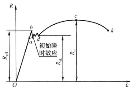
图 1-2 应力-应变曲线
