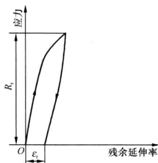
图 1-3 规定残余延伸强度
