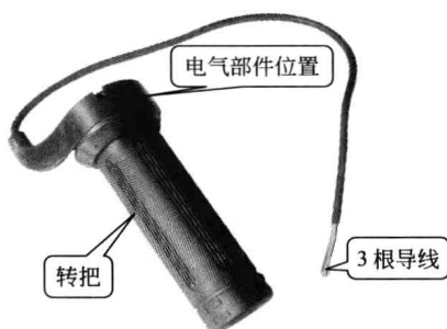
图 1-13 普通调速转把的外形
