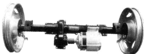
(b) BL-Z 双驱差速后桥总成
