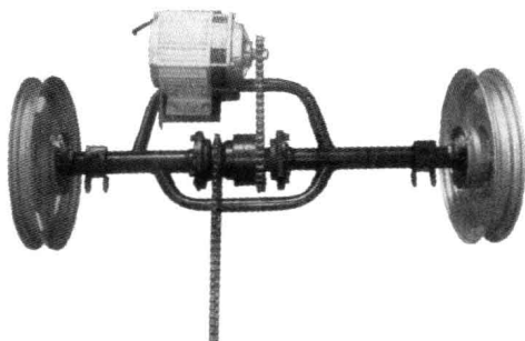
(c) 双链双驱动叉速后驱动桥
