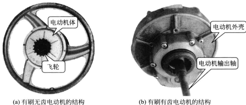
图 1-5 有刷电动机的结构
