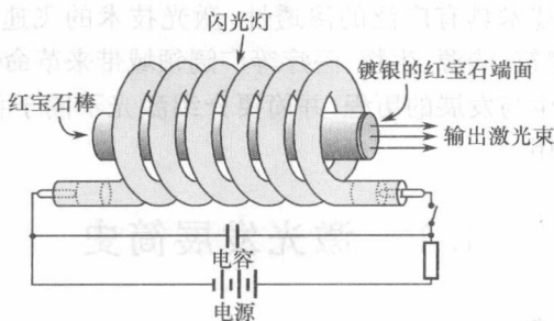
图 1-1 世界上第一台红宝石激光器的结构
