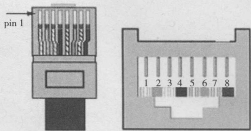
图 1-1 RJ-45 连接器
