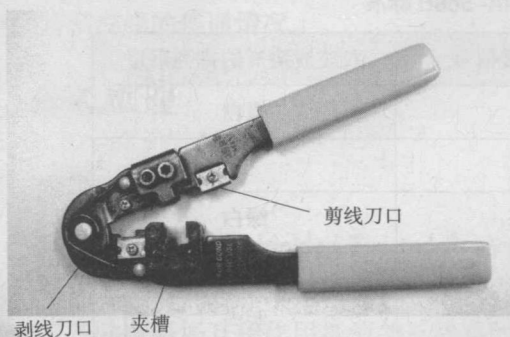
图 1-2 网线钳
