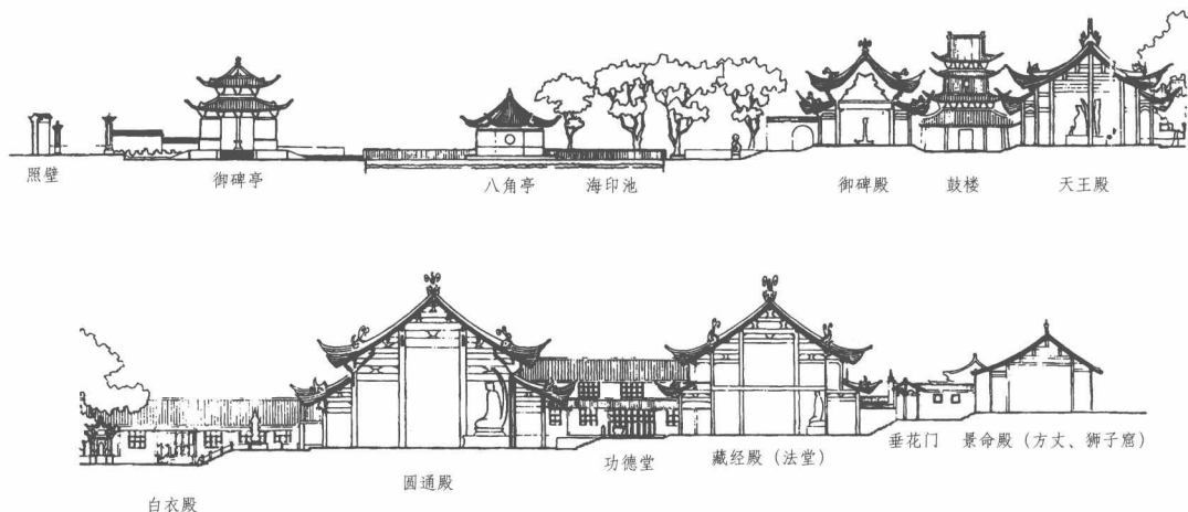
图1 清代重建普济禅寺纵剖面图 〔二〕
