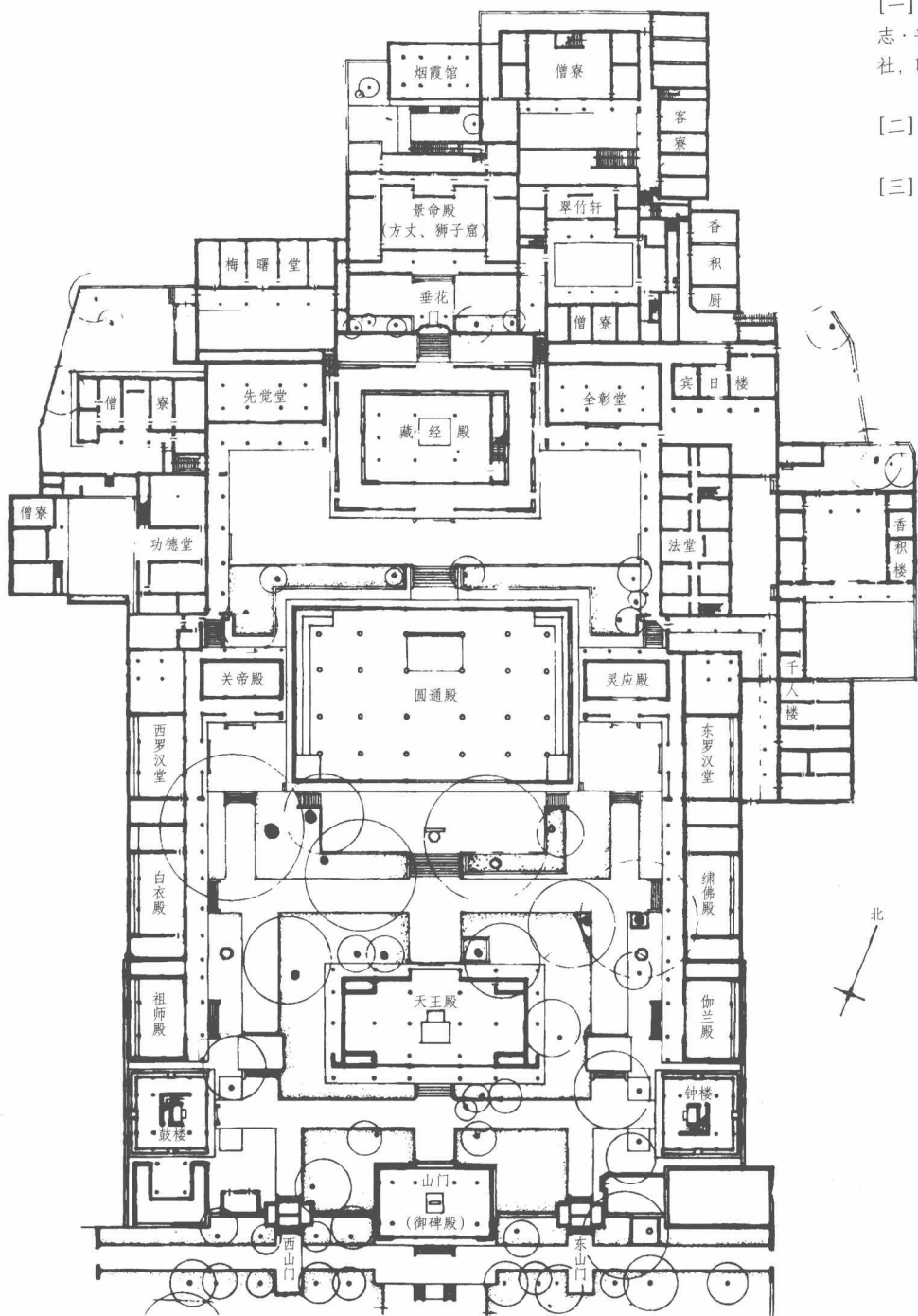
图2 清代重建普济禅寺平面图 [三]
