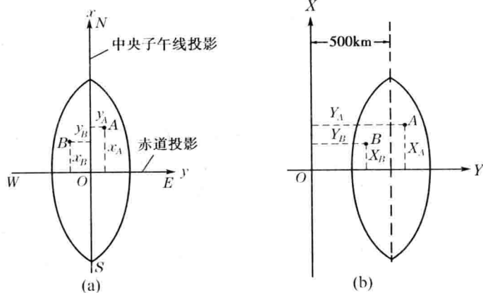
图 1-5 高斯平面直角坐标
