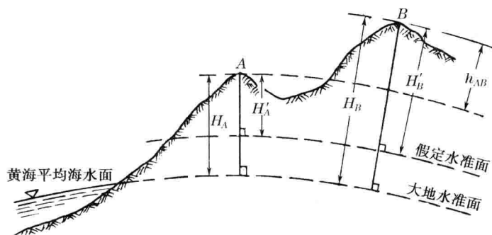
图 1-7 高程和高差
