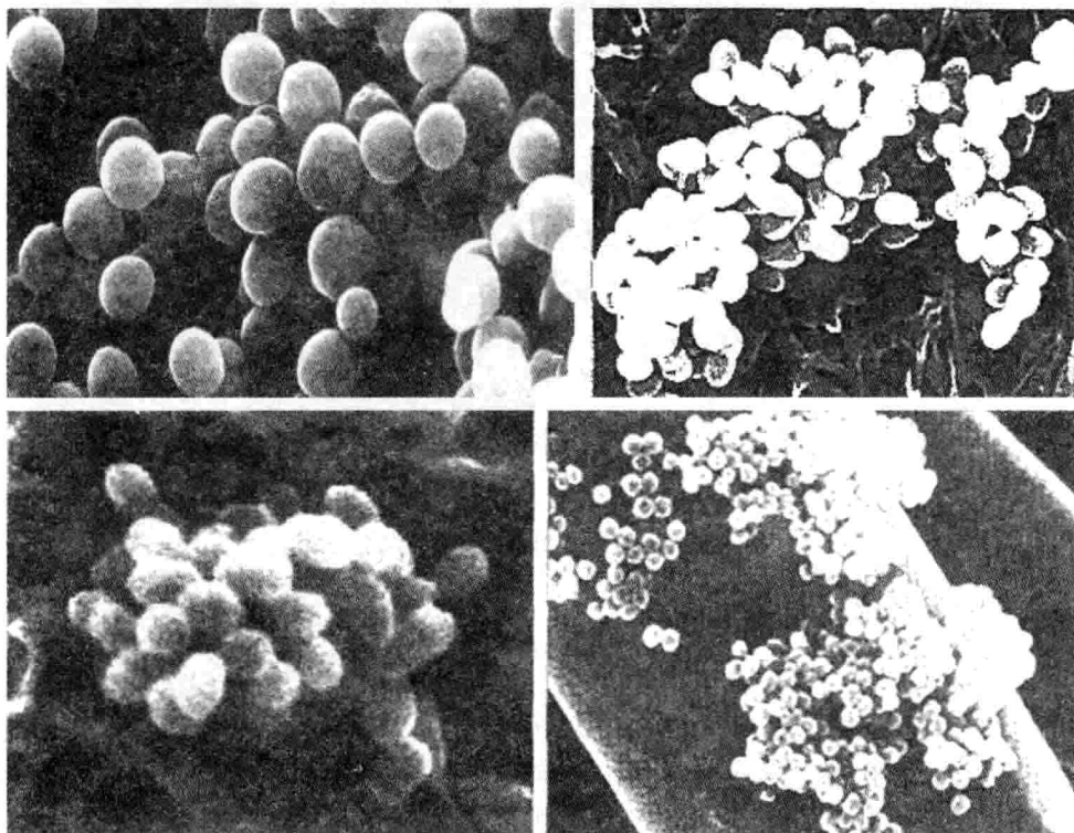
图 1.4 葡萄球菌
