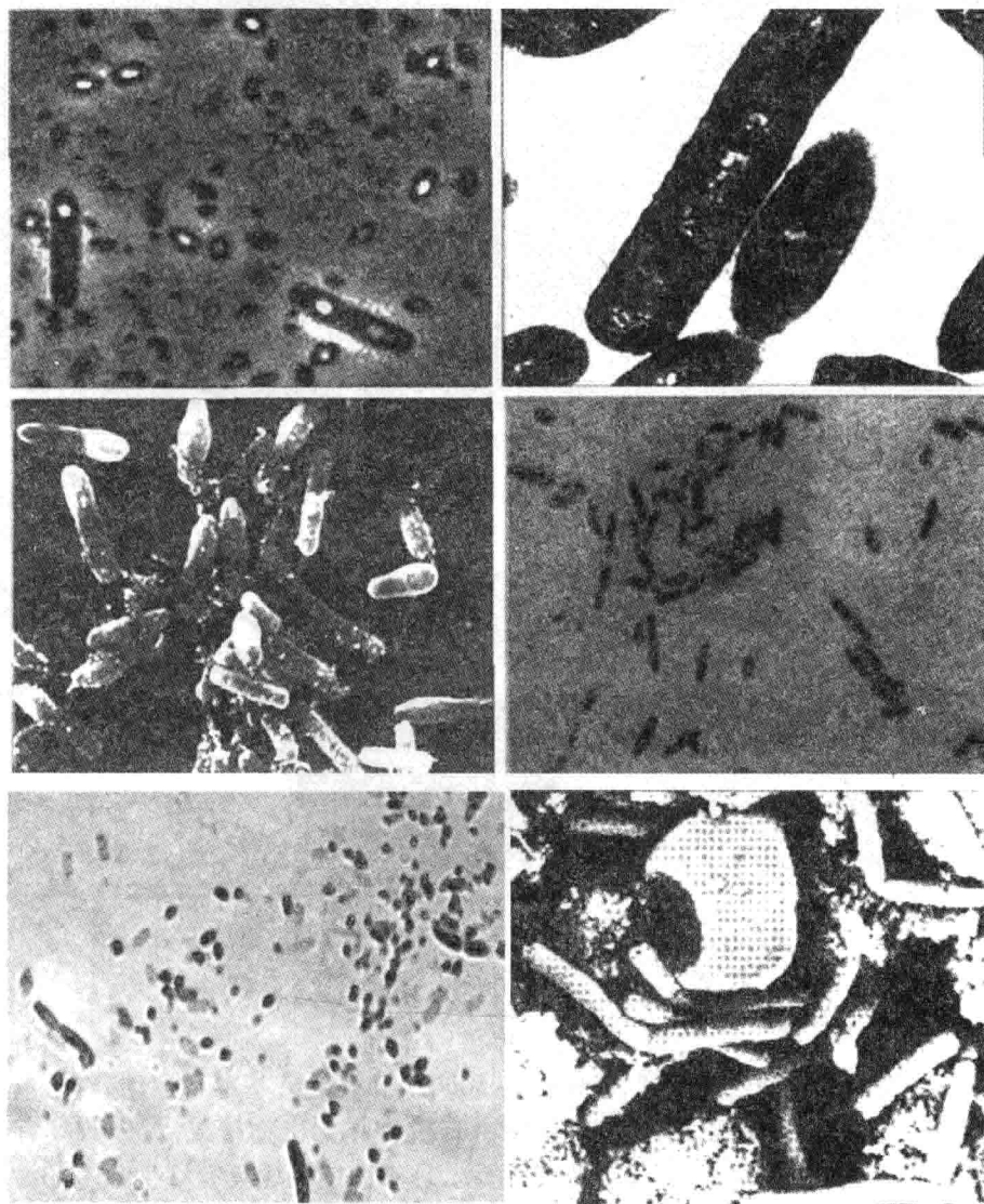
图 1.11 芽孢杆菌属
