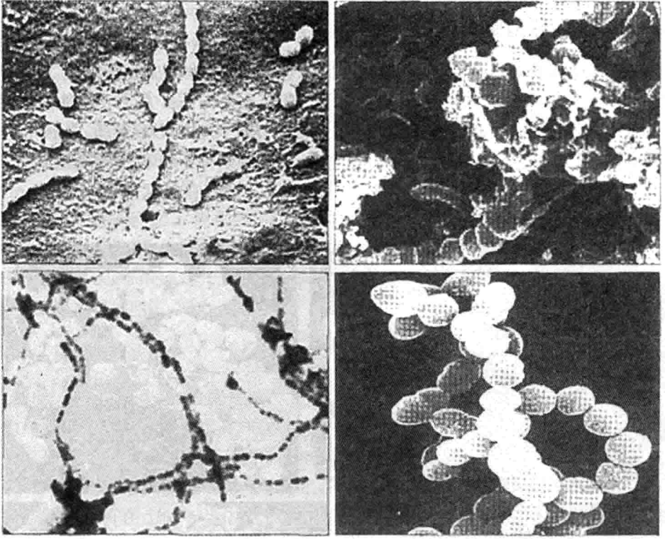
图 1.5 链球菌
