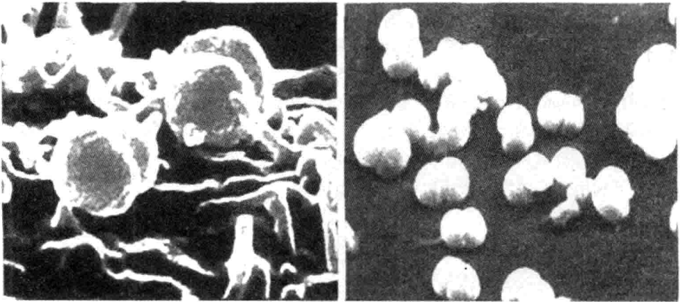
图 1.6 奈瑟菌属
