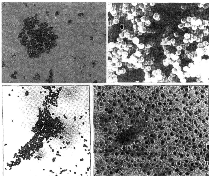
图 1.3 微球菌
