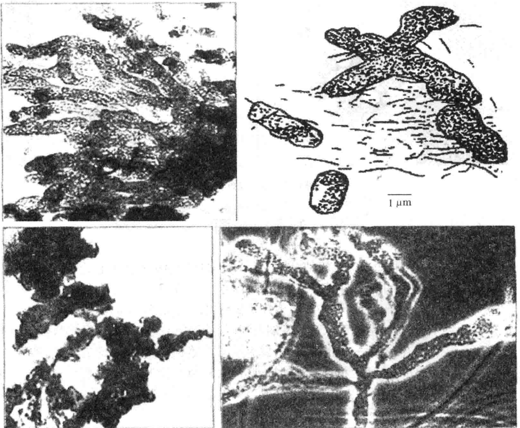
图 1.10 动胶菌属
