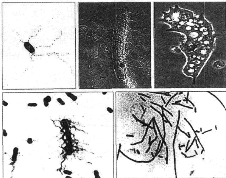
图 1.14 变形杆菌属
