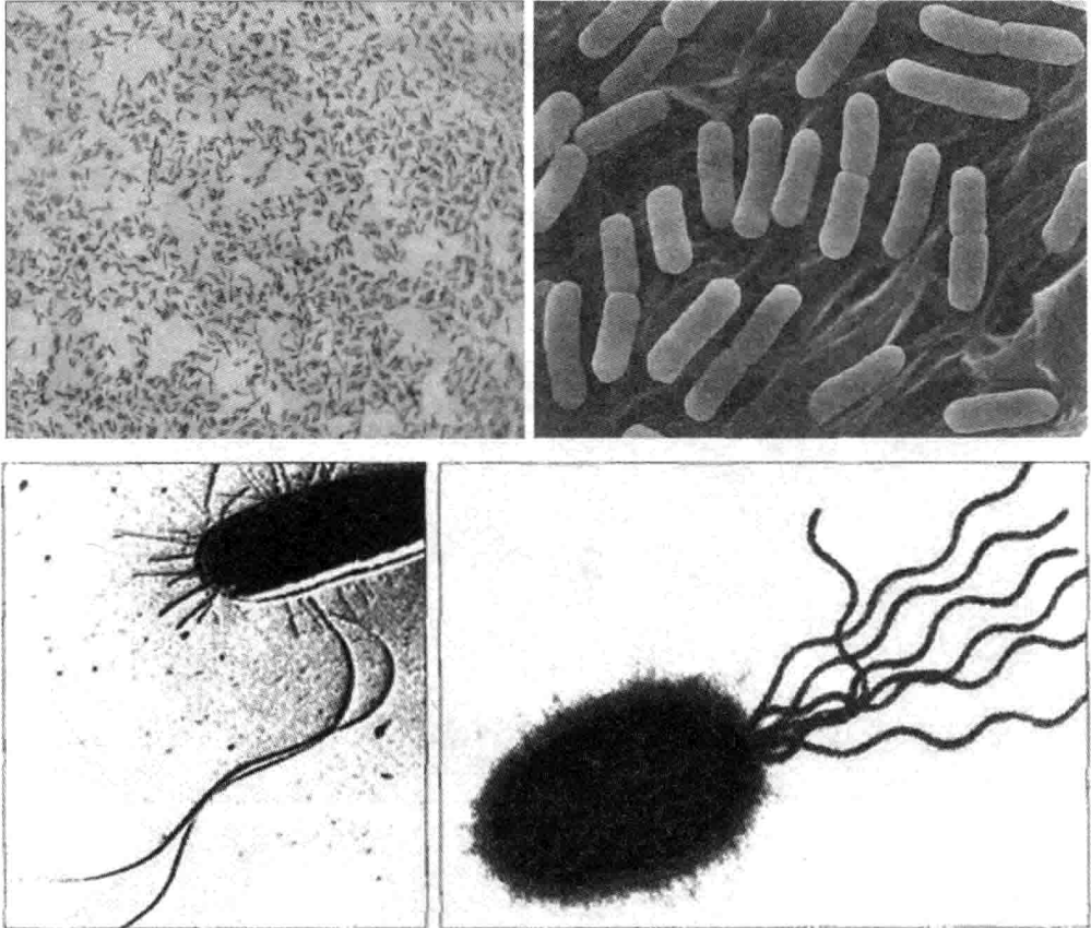
图 1.12 埃希菌属
