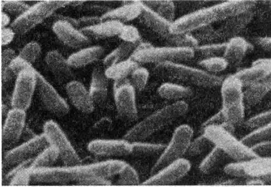
图 1.8 杆菌
