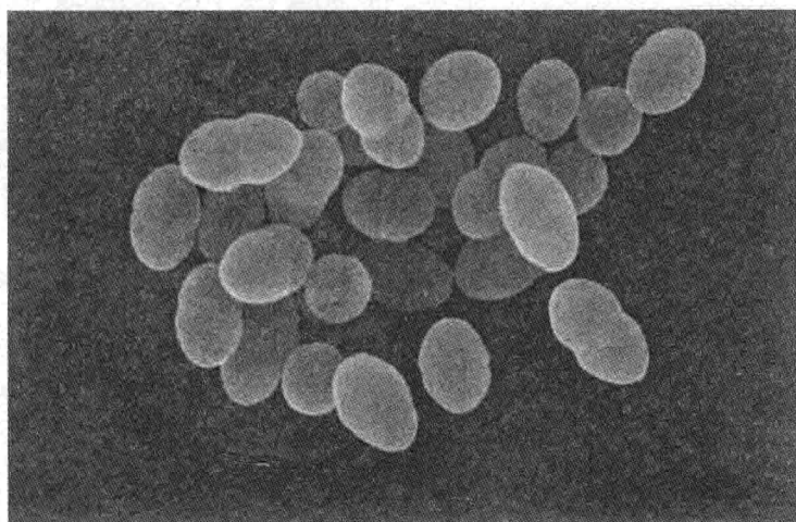
图 1.1 球菌
