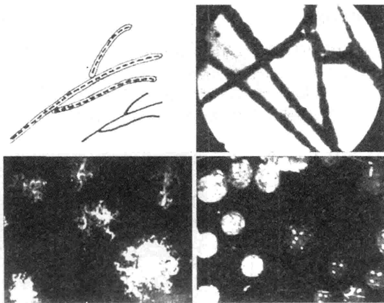
图 1.13 球衣菌属
