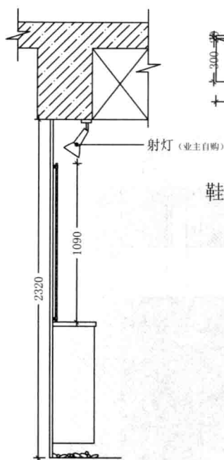
鞋柜方案2鞋柜兼屏风侧面图
