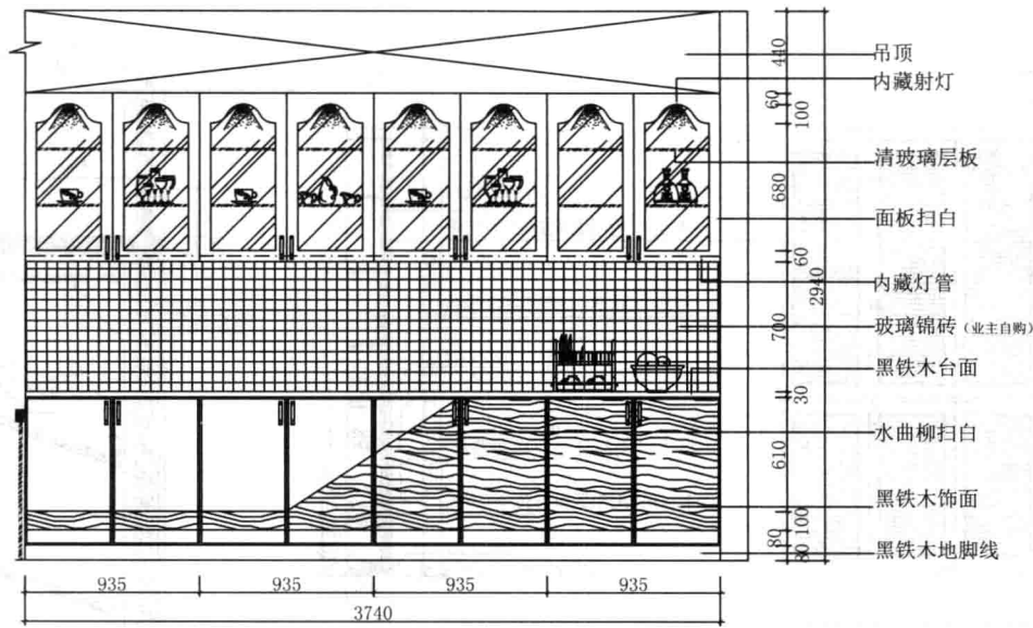
酒柜方案1立面图
