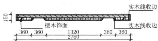
柜子方案1柜门大样图
