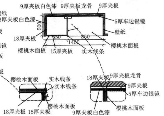
柜子方案2剖面图B
