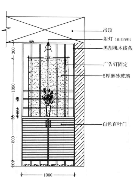
鞋柜方案2鞋柜兼屏风立面图
