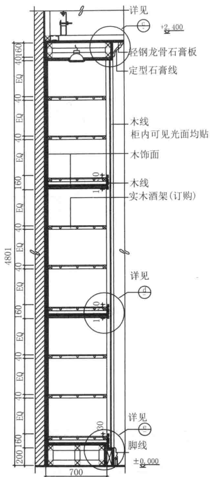
酒柜方案2大样图b
