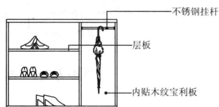
鞋柜方案3鞋柜内部结构图
