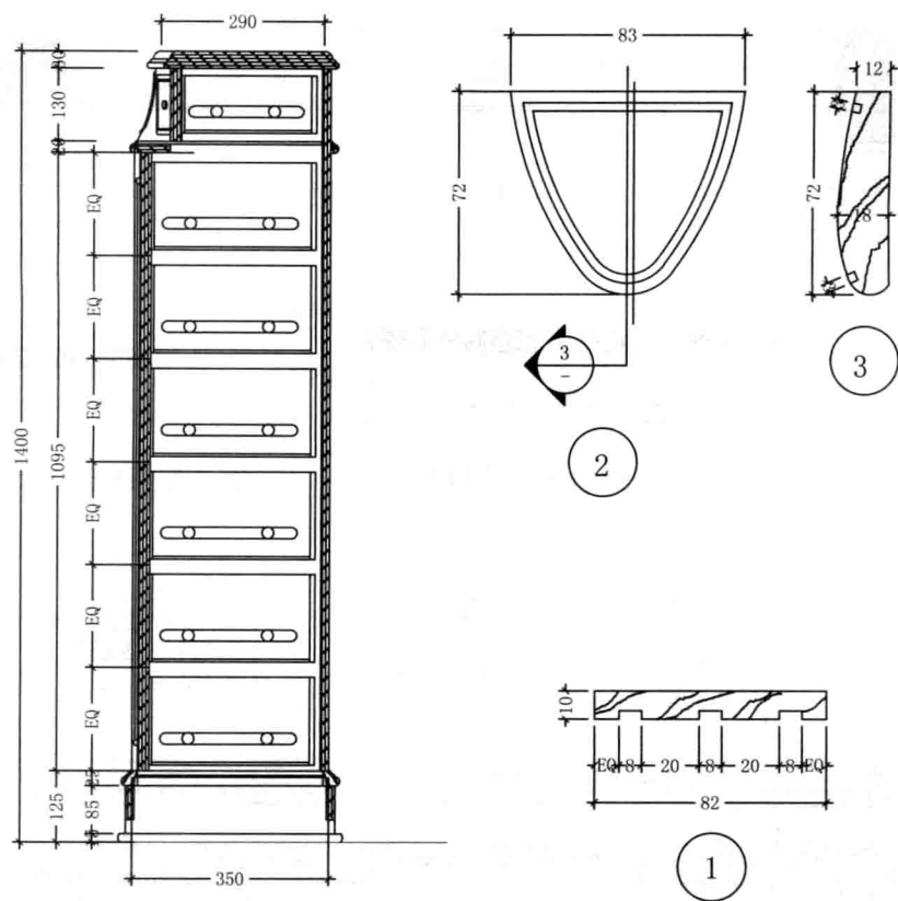
鞋柜方案4侧剖面图
