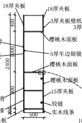
柜子方案2剖面图A
