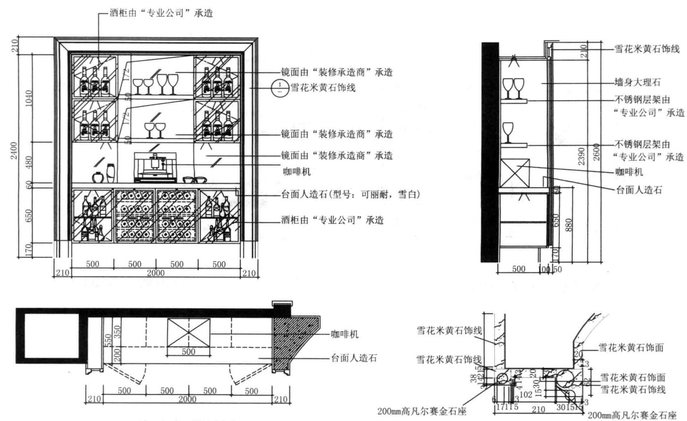
酒柜方案1设计图
