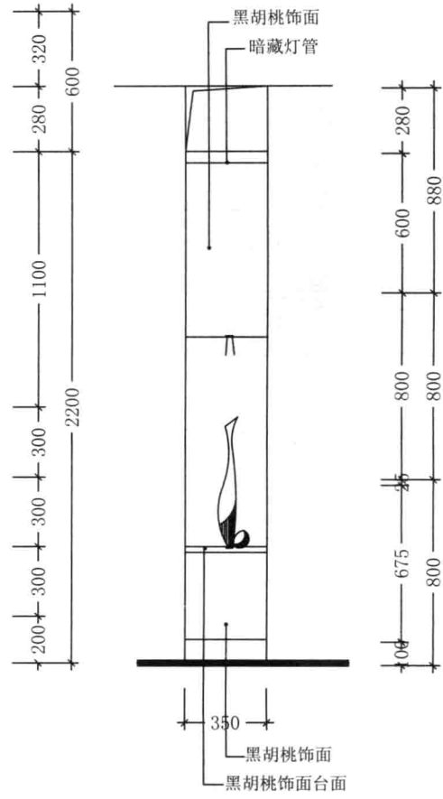
鞋柜方案1侧立面图
