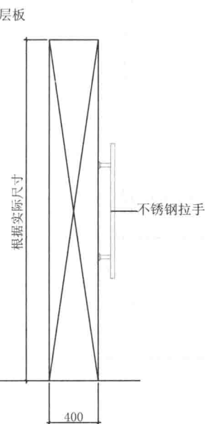
酒柜方案2侧立面图
