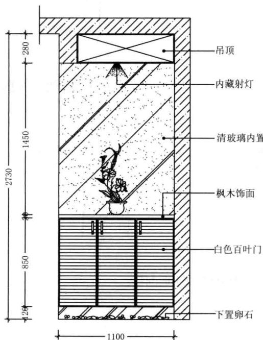
鞋柜方案3鞋柜立面图
