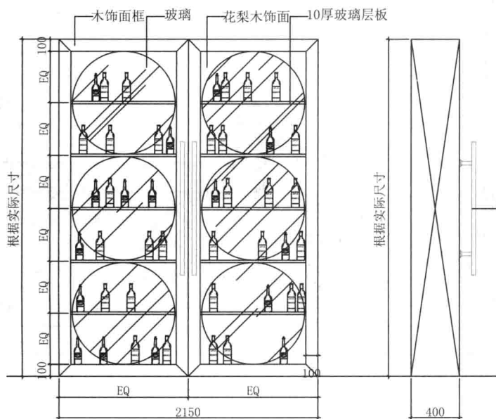
酒柜方案2正立面图
