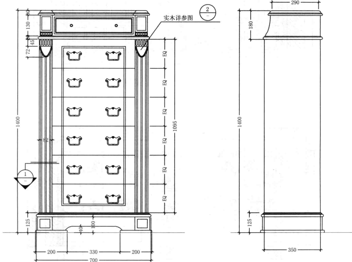
鞋柜方案4正立面图
