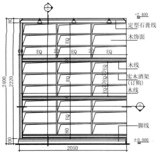
酒柜方案2立面图
