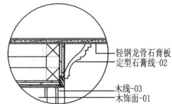
酒柜方案2大样图c
