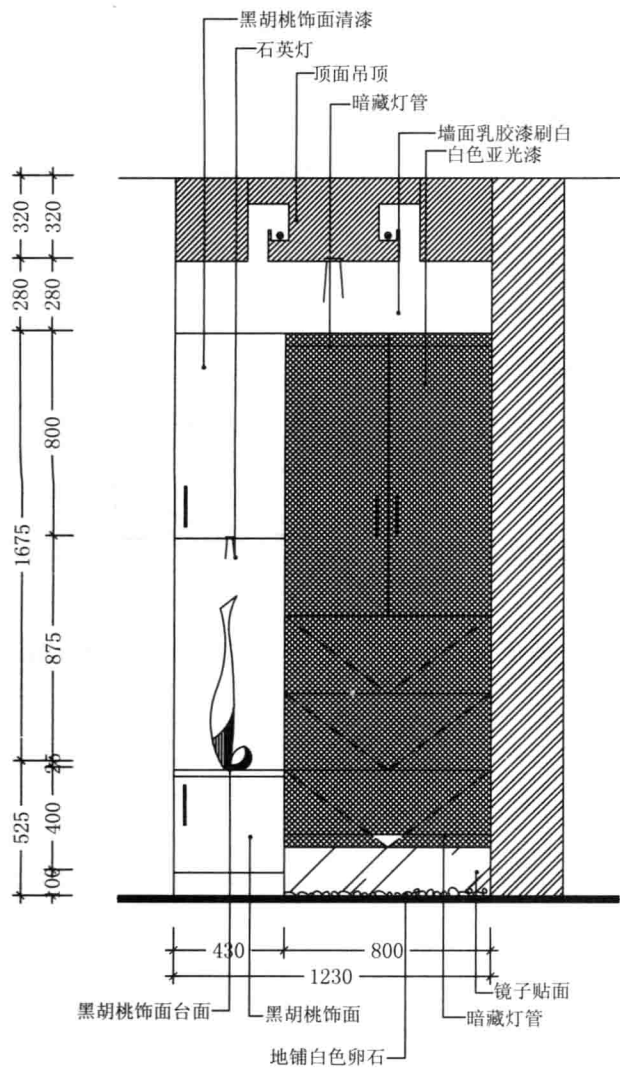
鞋柜方案1立面图
