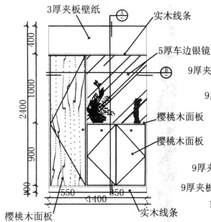
柜子方案2柜子立面图
