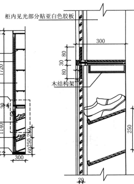
柜子方案3大样图
