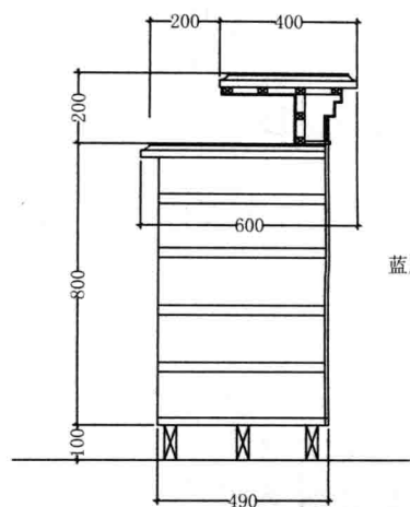
吧台方案1剖面图A
