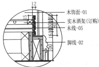
酒柜方案2大样图e
