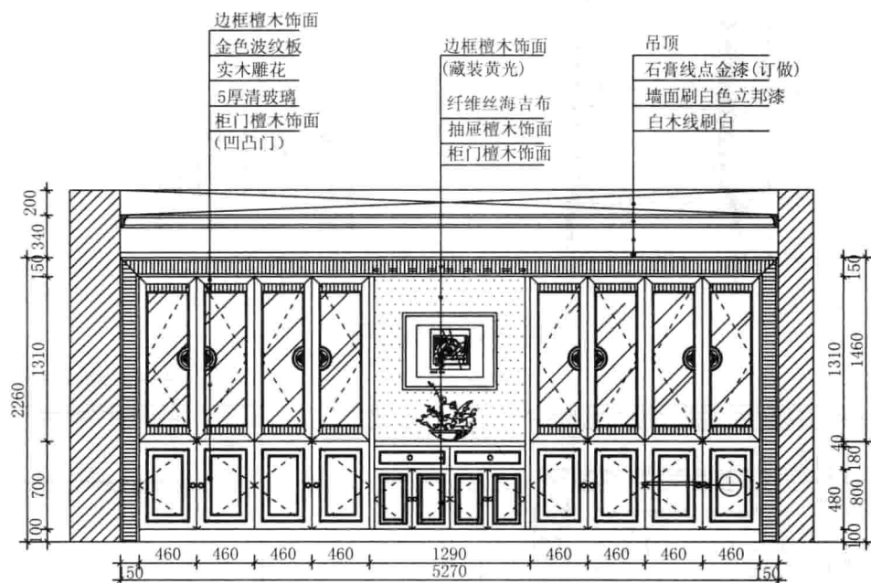
柜子方案1壁柜立面图
