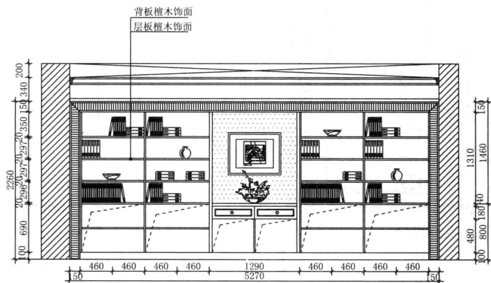
柜子方案1壁柜立面图
