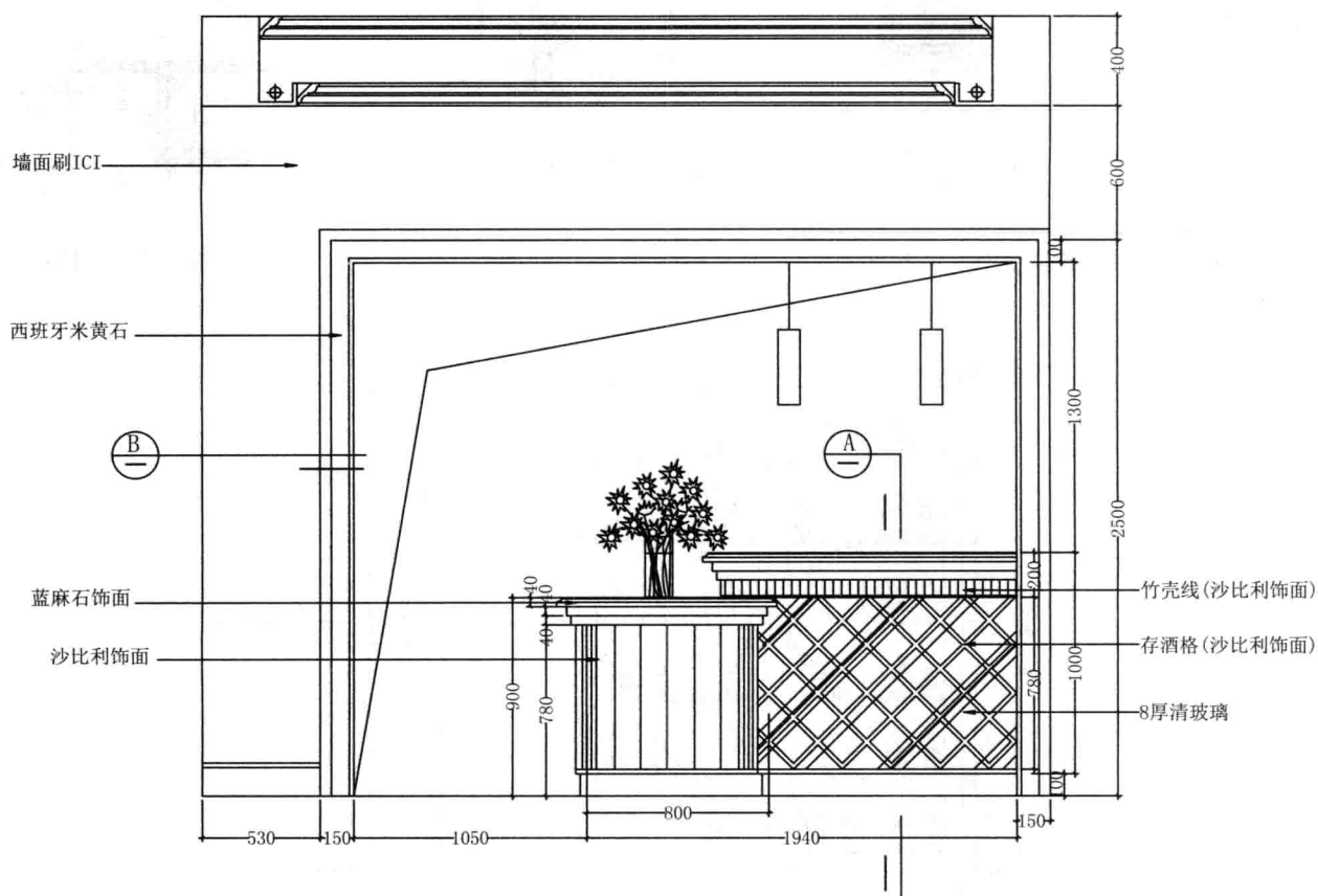
吧台方案1立面图
