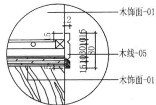
酒柜方案2大样图d
