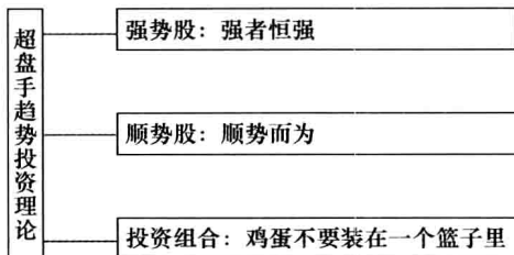
图 1.1 超盘手趋势投资理论框架图
