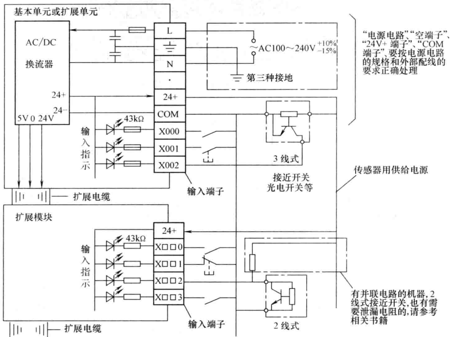
图 1-11 输入器件的接线示意图
