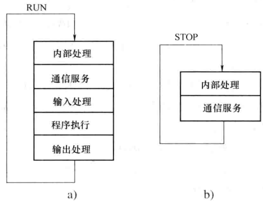
图 1-2 PLC 的基本工作模式
