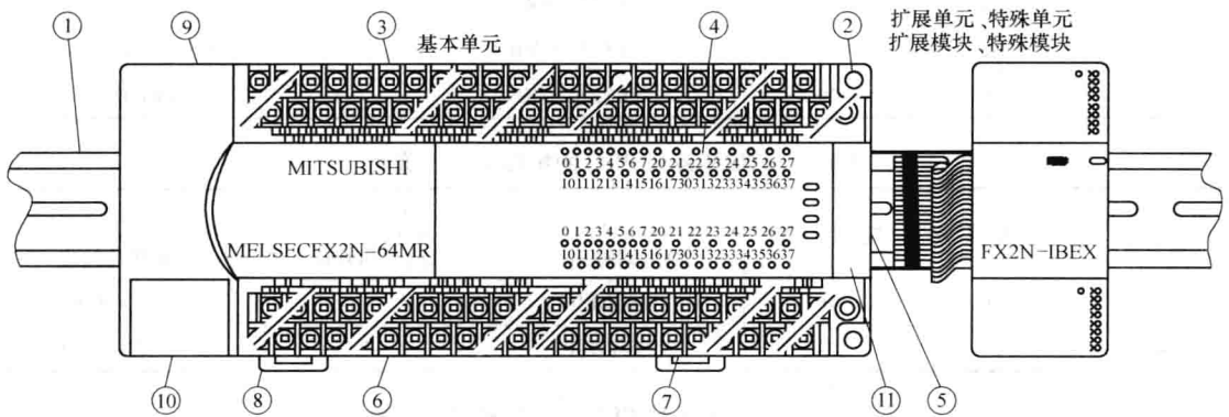
图 1-8 FX2N 机及扩展设备在 DIN 导轨上的安装示意图
