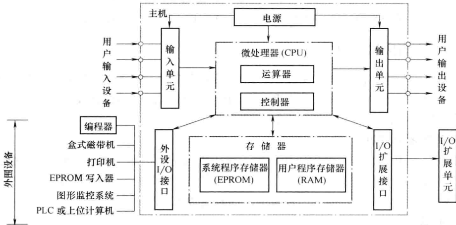
图 1-1 PLC 硬件系统的组成框图
