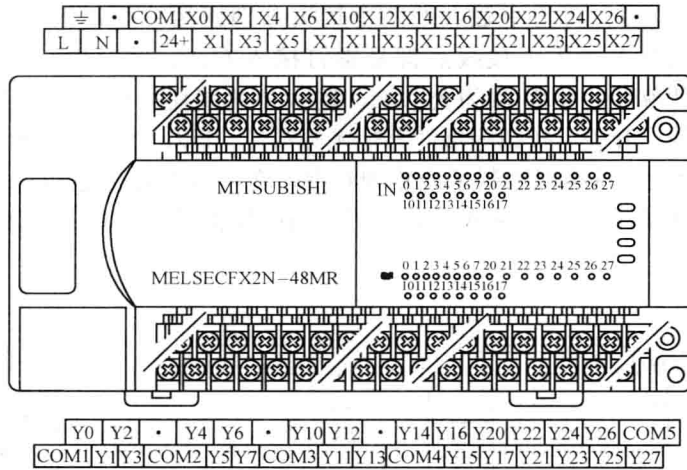
图 1-9 FX2N-48M 的接线端子排列图
