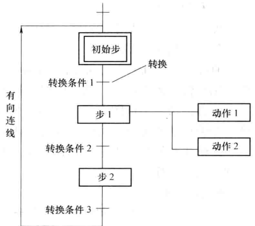
图 1-5 顺序功能图
