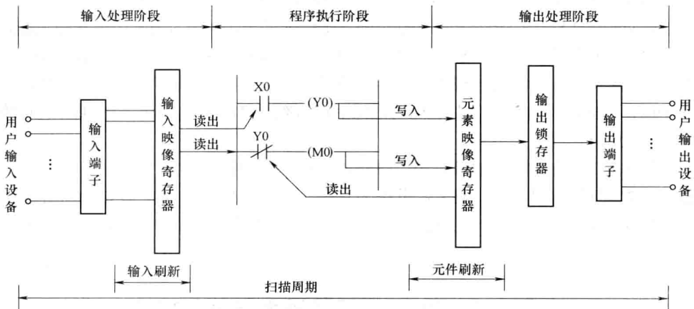
图 1-3 PLC 的工作过程
