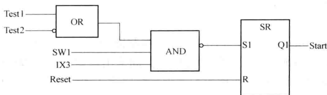
图 1-6 功能块图
