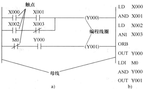
图 1-4 梯形图和对应的指令表
