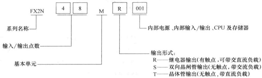
图 1-7 基本单元型号名称及其含义说明
