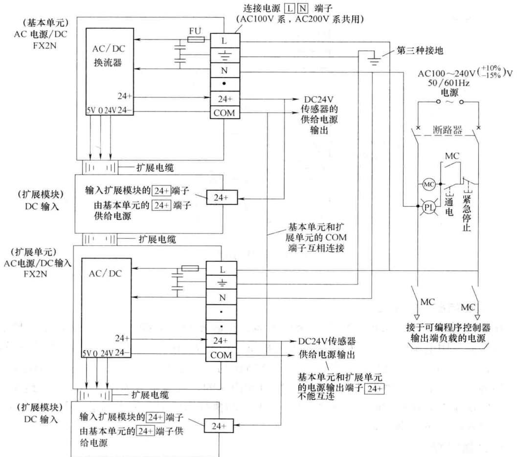
图 1-10 基本单元接有扩展模块时交直流电源的配线示意图
