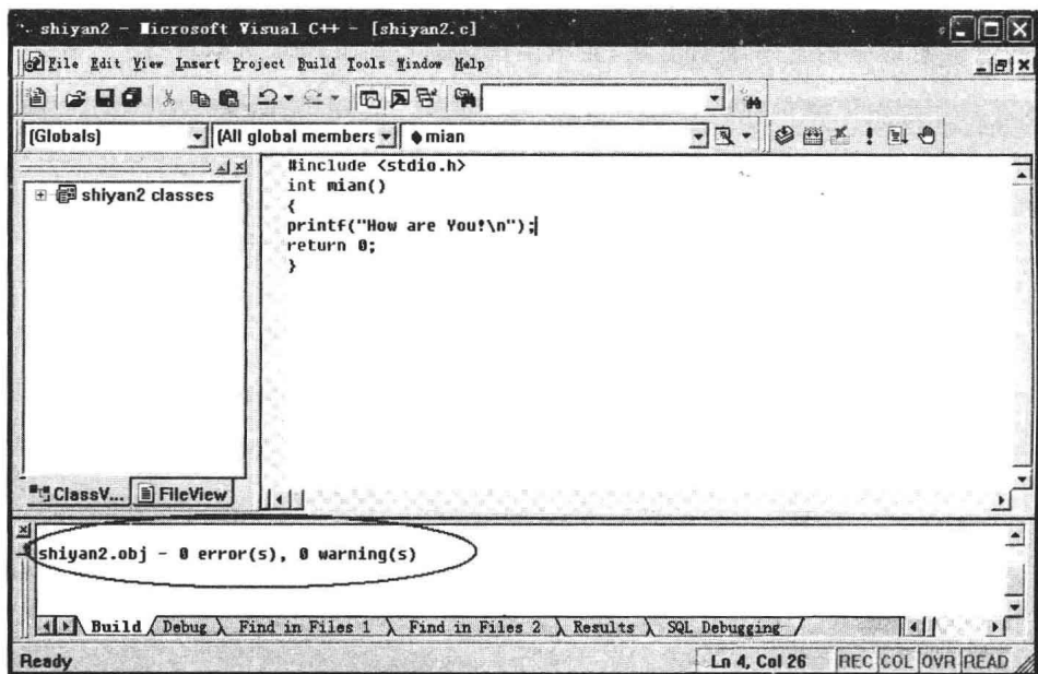
图 1-16 编译成功
