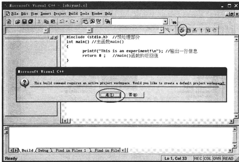
图 1-5 编译源程序
