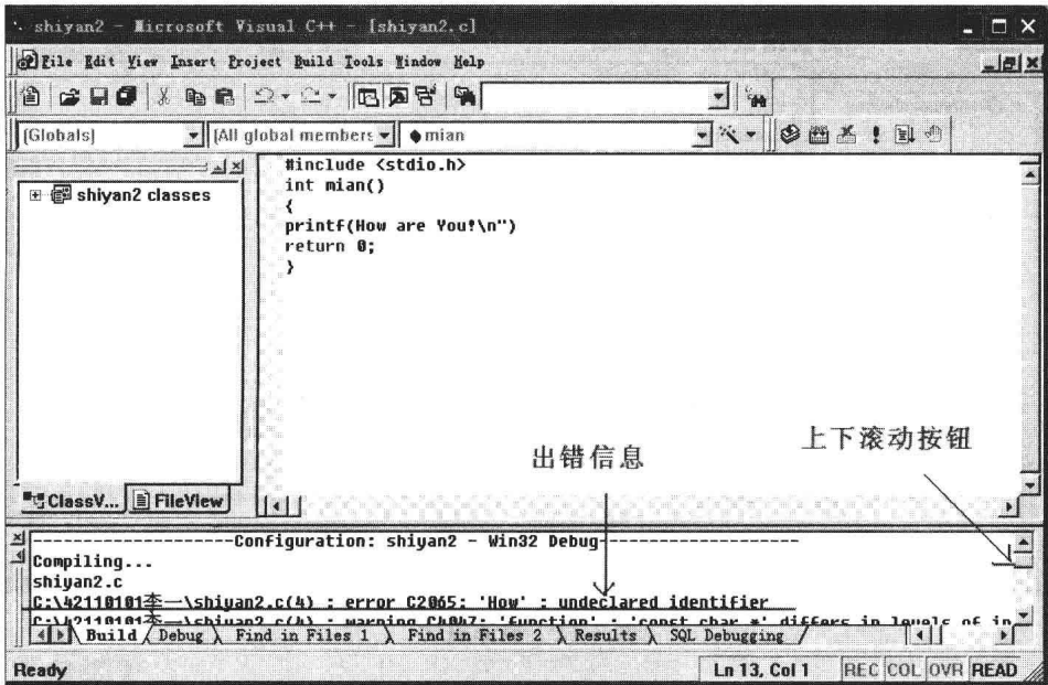
图 1-14 出错信息
